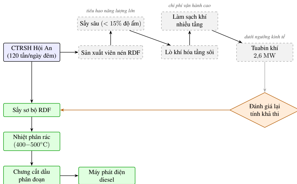
Hình 2.4: Chuyển đổi công nghệ xử lý CTRSH Hội An từ khí hóa sang nhiệt phân
