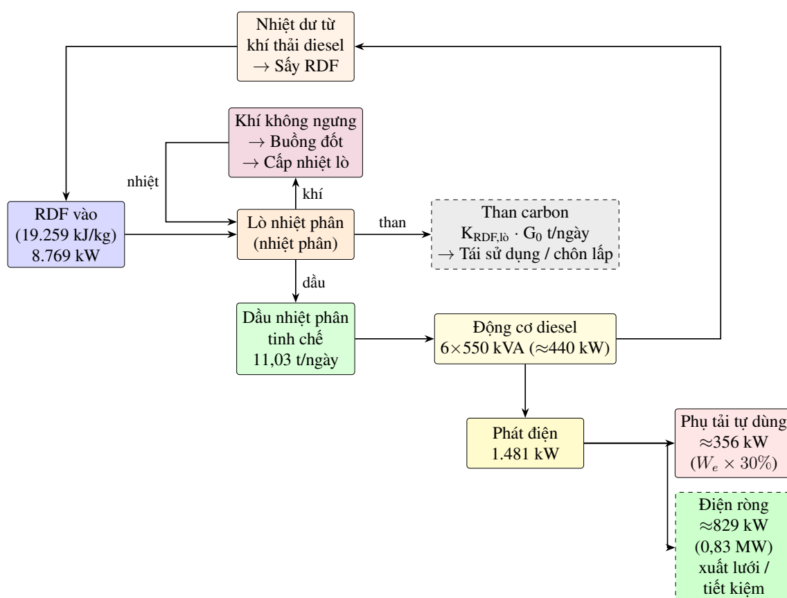
Hình 3.5: Sơ đồ tích hợp dòng năng lượng trong nhà máy
