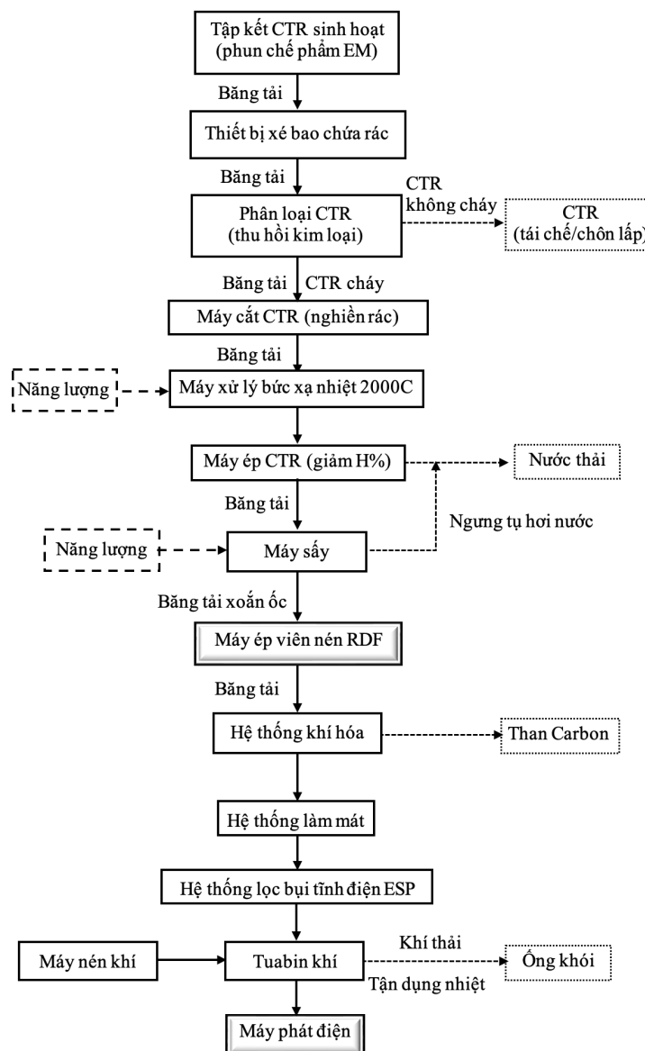
Hình 1.10: Sơ đồ khái quát phương án công nghệ khí hóa – tuabin khí ban đầu
