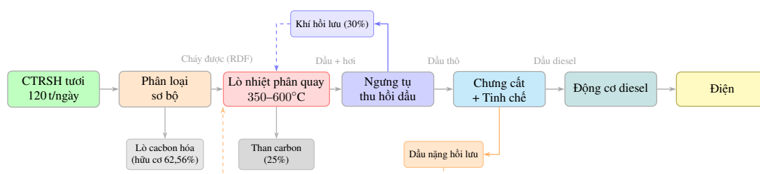
Hình 2.5: Sơ đồ công nghệ tổng thể: tiền xử lý – nhiệt phân – tinh chế – phát điện
