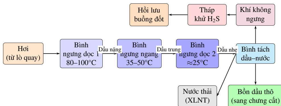
Hình 2.4: Sơ đồ hệ thống ngưng tụ thu hồi dầu ba cấp
