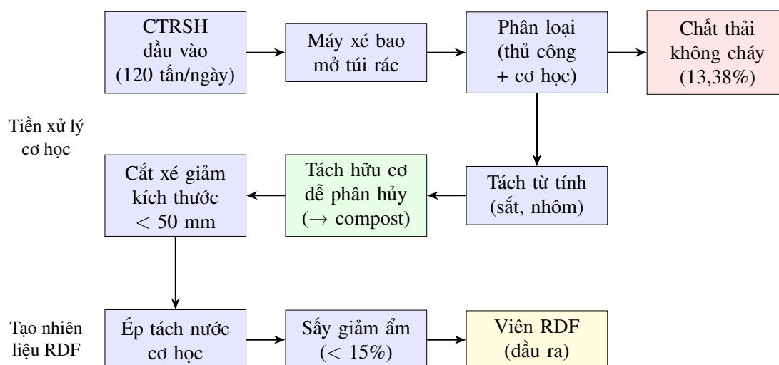
Hình 2.1: Sơ đồ nguyên lý hệ thống tiền xử lý và tạo viên nhiên liệu RDF
