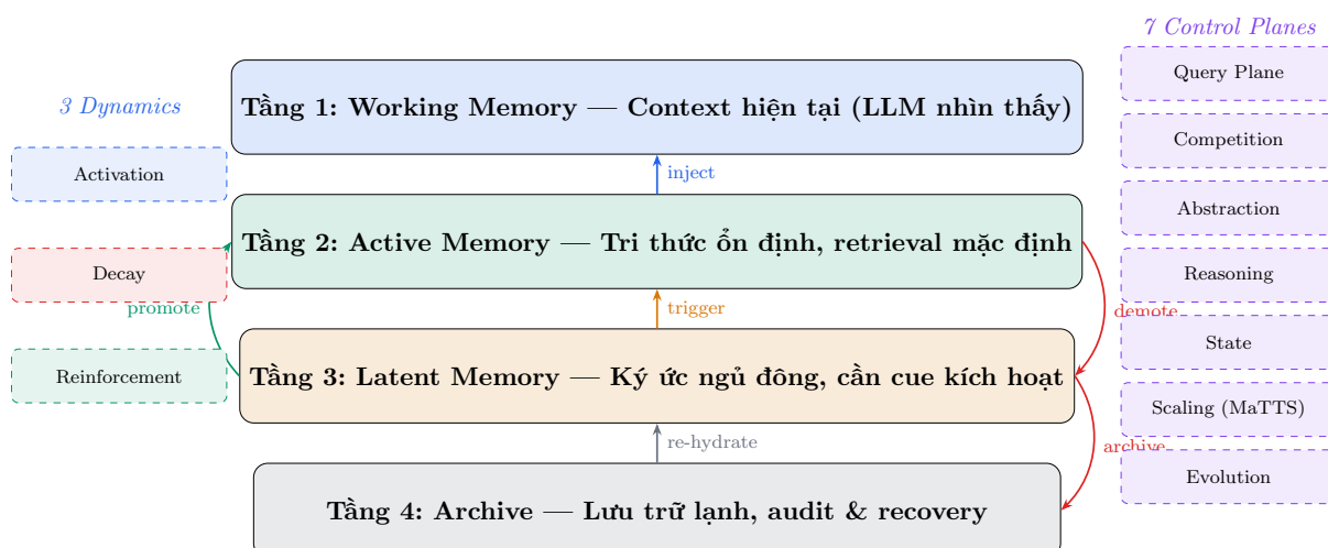
Hình 1: Kiến trúc tổng thể TAM: 4 tầng lưu trữ + 3 cơ chế động lực học + 7 lớp điều phối ngang.
