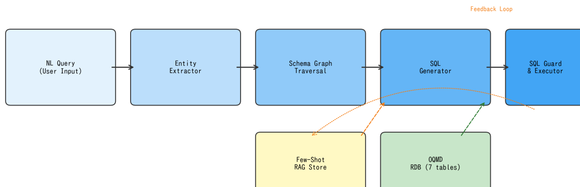
Figure 1: Schema Graph 支援 Text-to-SQL パイプラインのシステムアーキテクチャ。実線矢印は主要データフロー、破線矢印は Few-Shot RAG フィードバックループ（成功したクエリペアが蓄積・検索される）を示す。SQL ガードはデータベース実行前の最終安全層として機能する。
