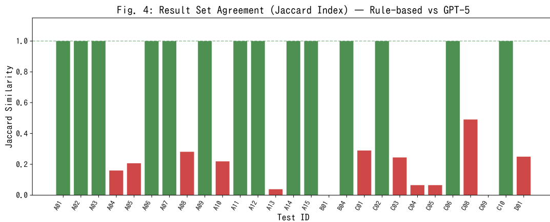
Figure 4: Rule-based と GPT-5 結果セット間の Jaccard 指数。緑 : \geq 0.8 (高一致)、橙 : 0.5\text{--}0.8 (中程度)、赤 : < 0.5 (低)。低一致ケースは主に GPT-5 の優れた意味理解に起因 (例 : B01: Xe 化合物、C09: NiAl 特定)。
