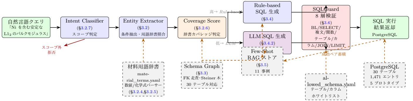
Figure 2: システムアーキテクチャの全体構成。実線矢印は主要データフロー、破線矢印（橙色）はデータ参照・フィードバックループを示す。Coverage Score に基づき Rule-based（高カバレッジ）または LLM（低カバレッジ）経路に岐分し、いずれも Schema Graph（30 テーブル FK 走査）による JOIN パス制約と SQLGuard 8 層検証を経て安全な SQL が生成・実行される。成功したクエリペアは Few-Shot RAG ストアに蓄積され、以降の LLM 生成に活用される。
