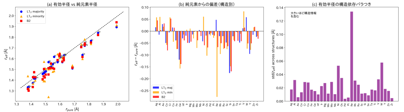
Figure 11: L1 2 構造における構造依存有効半径。多数派サイト（面心、配位殻: 同種 8 + 異種 4）の有効半径偏差 \langle |\Delta r_{maj}| \rangle = 0.036 Å に対し、少数派サイト（頂点、配位殻: 異種 12）は \langle |\Delta r_{min}| \rangle = 0.045 Å と約 25%大きい。完全異種配位殻をもつ少数派原子は周囲の化学環境の影響を最も強く受け、純元素半径からの乖離が大きい。
