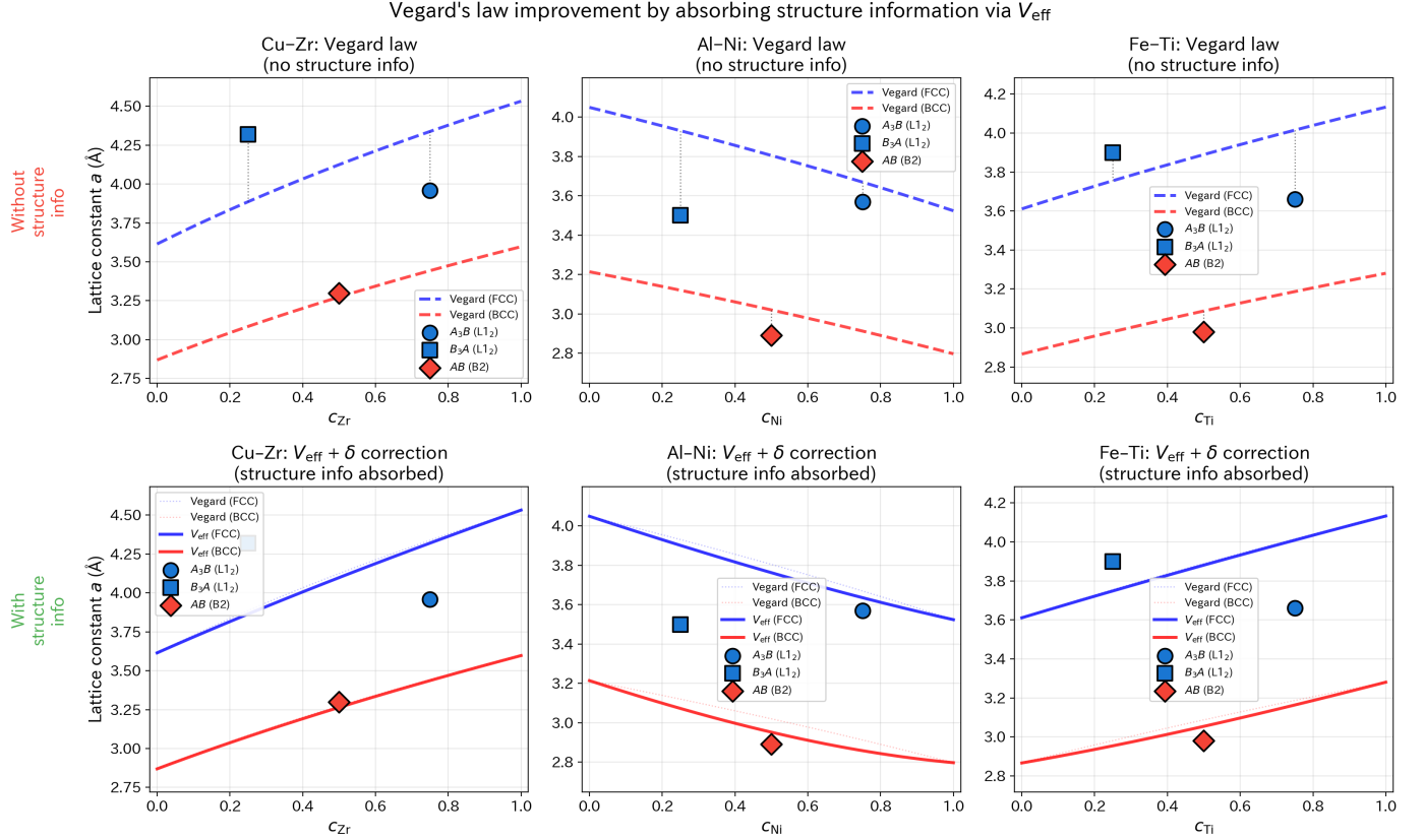
Figure 14: 構造情報吸収による Vegard 則の改善（代表 3 ペア：Cu-Zr, Al-Ni, Fe-Ti）。上段：Vegard 則（純元素体積の線形補間）。赤破線：BCC 予測、青破線：FCC 予測。DFT 計算値（丸： A_3B L1_2 、四角： B_3A L1_2 、菱形： AB B2 ）は Vegard 直線から系統的に偏差する。下段： V_{\text{eff}} ( \delta^{(s)} 補正後)。赤実線：BCC ( \delta^{B2} 使用)、青実線：FCC ( \delta^{L1_2} 使用)。構造特異的な \delta 補正により Vegard 直線が曲線に変換され、DFT 点に接近する。薄い点線は補正前の Vegard 則。
