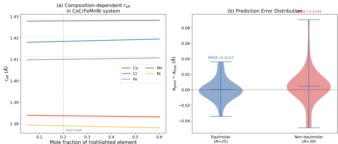
Figure 13: 組成依存有効半径 r_{eff} の振る舞い。(a) CoCrFeMnNi (Cantor 合金) 系 FCC 合金における各元素の r_{eff} の組成依存性。1 成分の分率 c_i を 0.05–0.60 まで変化させ、残り 4 成分は均等配分。破線は純元素半径 r_{pure} 。正の \delta を持つ Mn の分率増加は周囲への膨張効果を増大させ、負の \delta を持つ Ni では逆の効果。等モル点 c_i = 0.2 付近で非線形応答が顕著。(b) 等モル ( N = 25 ) vs 非等モル ( N = 39 ) HEA の予測誤差分布。
