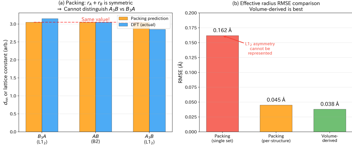
Figure 9: パッキング制約半径の解析。パッキングモデル ( d_{nn} = r_A + r_B ) で推定した半径による格子定数予測と実際の DFT 格子定数の比較。単一半径セットでは r_A + r_B が対称操作であるため a(A_3B) = a(B_3A) を強制し、L1 2 の非対称性（平均差 0.328 Å）を表現できない。結果として RMSE = 0.162 Å と Vegard 則の 5 倍以上の残差が生じる。
