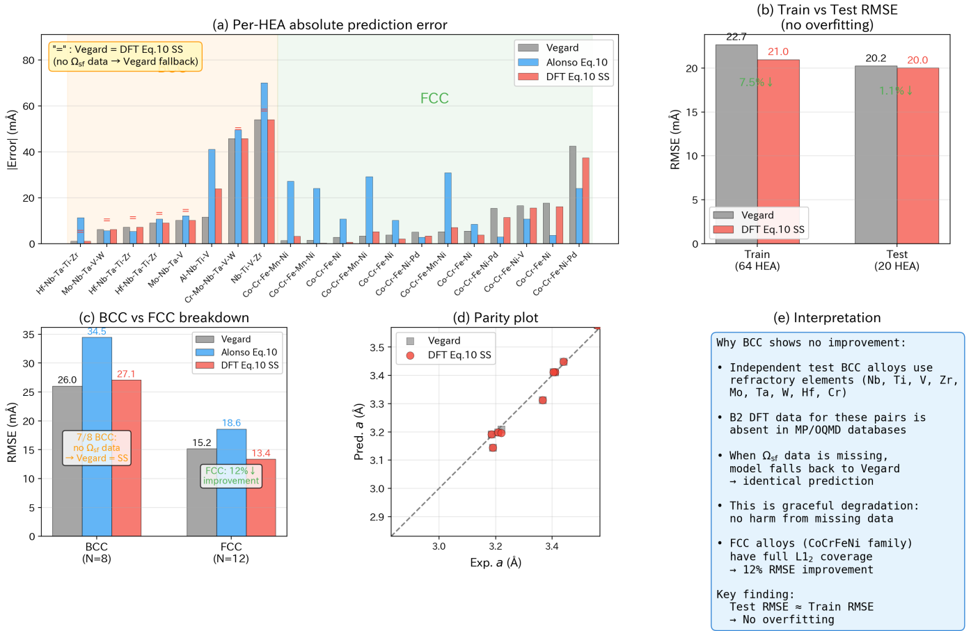
Figure 4: 独立テストセット検証の詳細 (20 HEA: BCC 8 個 + FCC 12 個)。(a) 各 HEA の絶対誤差 (mÅ 単位) の手法別比較。BCC 8 合金中 7 合金で Vegard と DFT Eq. 10 SS が完全一致 (“=” 印) : B2 DFT データ欠損による Vegard フォールバック。(b) 訓練・テスト間 RMSE 比較 : テスト RMSE \approx 訓練 RMSE (過学習なし)。(c) BCC/FCC 別 RMSE 分解 : 改善は L1_2 データカバレッジのある FCC に集中 (12%改善)。(d) パリティプロット。(e) BCC 改善が小さい構造的理由の説明。
