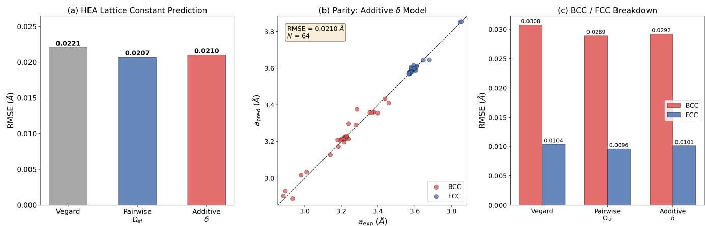
Figure 12: 加法分解 \delta^{(s)} モデルによる HEA 格子定数予測の可視化 (64 HEA)。(a) Vegard 則・ペアワイズ \Omega_{sf} ・加法 \delta^{(s)} の RMSE 比較棒グラフ。加法モデル (RMSE = 0.0210 Å) はペアワイズ (0.0207 Å) とほぼ同等。(b) パリティプロット (予測 vs 実験格子定数)。BCC/FCC 双方で系統的バイアスなし。破線は完全一致線。(c) BCC/FCC 構造別 RMSE 分解。FCC (0.0101 Å) が BCC (0.0292 Å) より高精度であるのはペアワイズモデルと共通の傾向。
