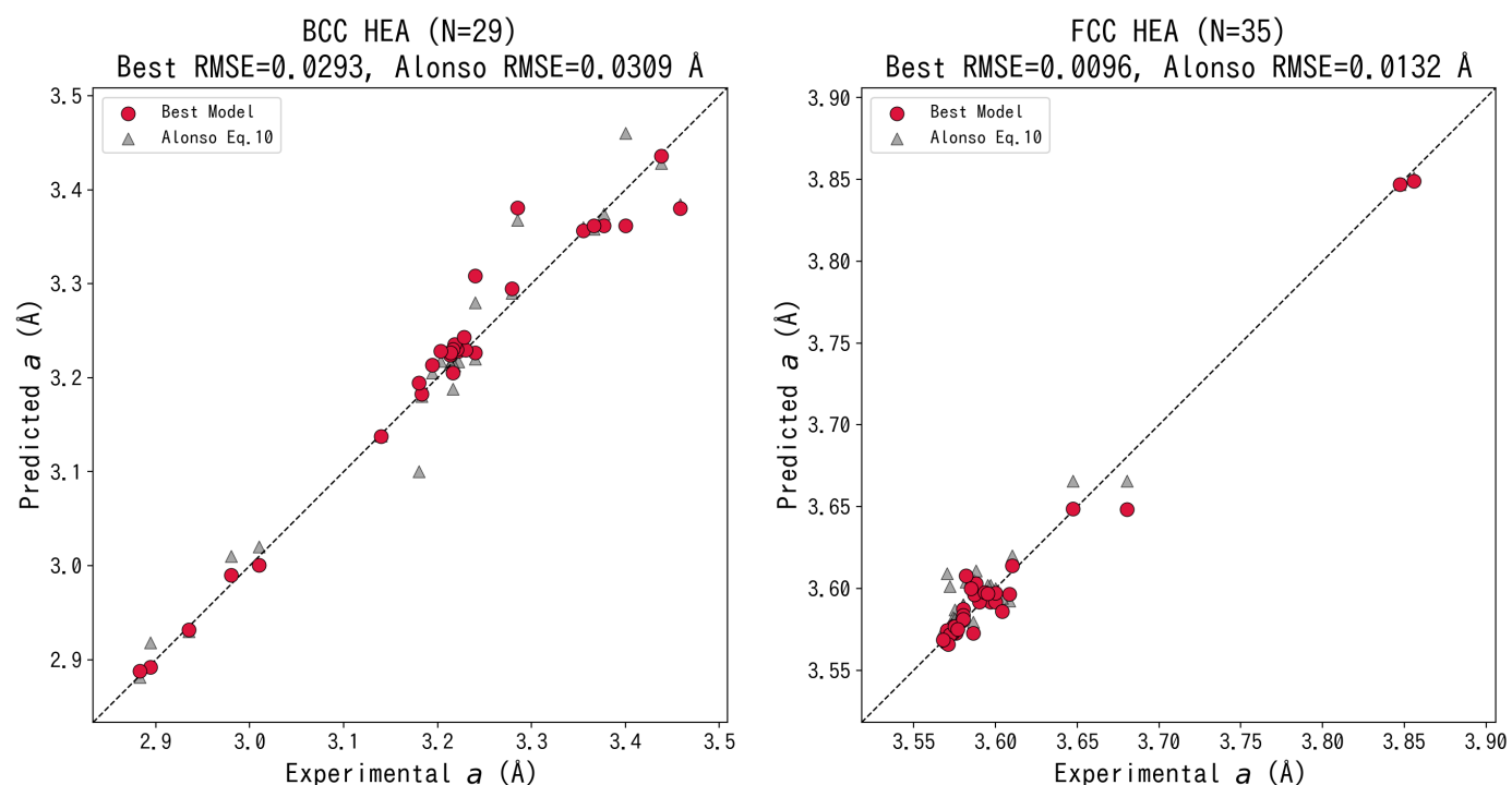
Figure 3: BCC (左、 N = 29 ) と FCC (右、 N = 35 ) 別のパリティプロット。FCC HEA (右) は DFT Eq. 10 SS で対角線にほぼ一致 (RMSE = 0.0096 Å)。BCC HEA (左) は格子定数範囲が広く ( a = 2.87\text{--}3.44 Å)、Al 含有合金で偏差がやや大きい。破線は完全一致線。
