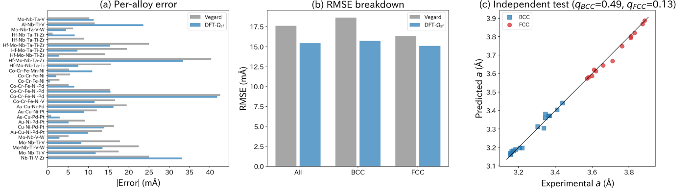
Figure 4: 独立テストセット (28 HEA、12 文献 18 元素) の予測性能。(a) 合金別絶対誤差。(b) 構造別 RMSE (灰: Vegard、青: DFT- \Omega_{sf} )。 (c) パリティプロット ( q_{BCC}=0.49 , q_{FCC}=0.13 )。BCC 15 合金 (青四角) と FCC 13 合金 (赤丸)。
