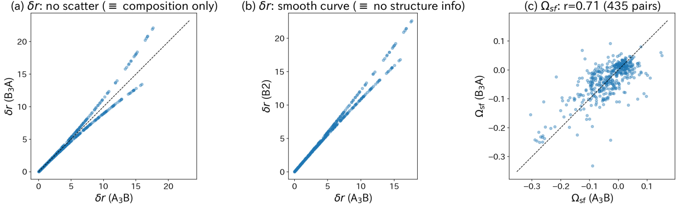
Figure A7: \delta r の構造不変性の検証 (435 ペア、4f 希土類+Y 除外後)。(a) \delta r(A_3B) vs \delta r(B_3A) : 完全一致 (構造情報ゼロ)。(b) \delta r(A_3B) vs \delta r(B2) : 滑らかな曲線 (組成のみの関数)。(c) \Omega_{sf}(A_3B) vs \Omega_{sf}(B_3A) : r = 0.71 (435 ペア)。対称でない散布は L1_2 の構造依存性を反映。
