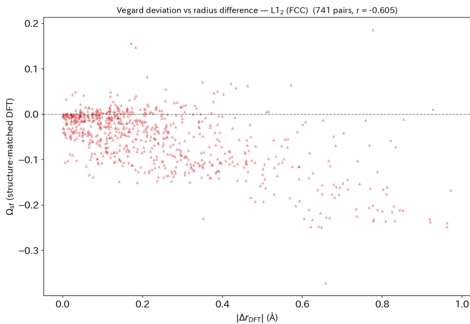
Figure A6: L1 2 \Omega_{sf} と純元素 DFT 半径差の関係 (741 ペア、 r = -0.61 )。B2 よりも強い負の相関を示し、サイズ差が大きいほど体積収縮が増大する。
