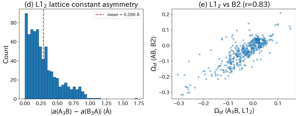
Figure A8: L1_2 構造の非対称性と構造間相関。(d) L1_2 格子定数差 |a(A_3B) - a(B_3A)| の分布 (754 ペア、平均 0.286 Å)。(e) L1_2 \Omega_{sf} vs B2 \Omega_{sf} (435 ペア、 r = 0.83 ) : 構造間で \Omega_{sf} は強い相関を持つが完全には一致しない。
