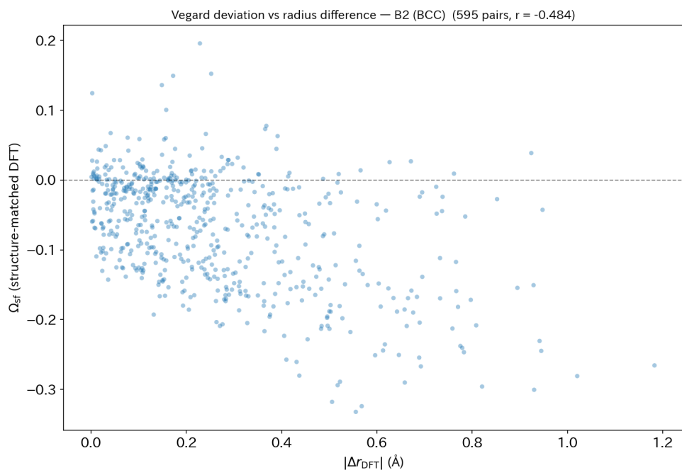
Figure A5: B2 \Omega_{sf} と純元素 DFT 半径差の関係 (595 ペア、 r = -0.48 )。半径差が大きいほど体積収縮（負の \Omega_{sf} ）が増大する傾向。
