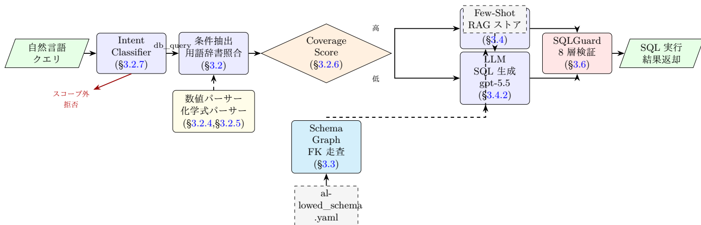
Figure 1: 提案手法の解析フロー全体図。自然言語クエリは Intent Classifier でスコープ判定後、用語辞書・数値/化学式パーサーで条件抽出される。Coverage Score に基づき Rule-based (高認識率) または LLM (低認識率) 経路に分岐し、いずれも Schema Graph (FK 走査) による JOIN パス制御と SQLGuard 8 層検証を経て安全な SQL が生成・実行される。破線矢印はデータ参照を示す。
