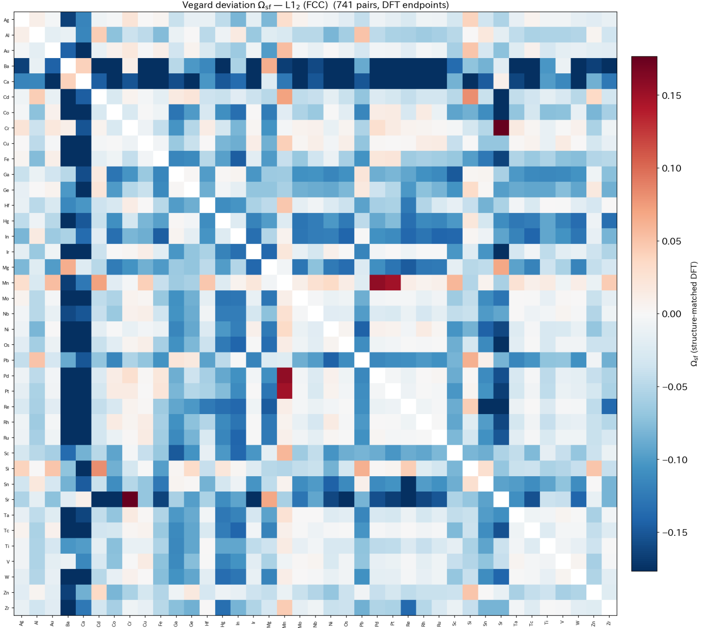
Figure A2: 全元素ペアの L1 2 (FCC 型) Ω sf ヒートマップ (741 ペア、39 元素、DFT 端点)。DFT L1 2 同種体積を端点とした Vegard 偏差。B2 より元素数が多く、A 3 B/B 3 A 非対称性が偏差の分散を広げる。
