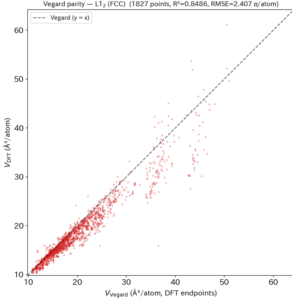
Figure A4: 全 L1_2 ペアの Vegard パリティプロット (1827 点、 R^2 = 0.849 、 RMSE = 2.407 \text{ Å}^3/\text{atom} )。4f 希土類+Y 除外後は、B2 と同程度の Vegard 則成立精度を示す。
