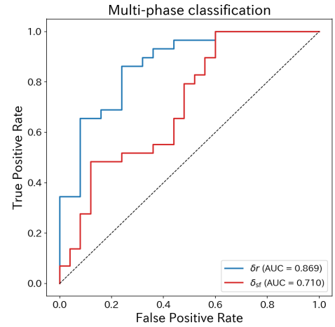
Figure A9: SS vs 非 SS 分類の ROC 曲線 (54 HEA)。 \delta r (AUC = 0.869) が \delta_{\text{sf}} (AUC = 0.710) を上回る。
