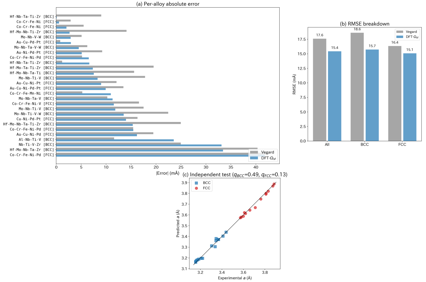
Figure 4: 独立テストセット（28 HEA、12 文献 18 元素）の予測性能。(a) 合金別絶対誤差。(b) 構造別 RMSE (灰: Vegard、青: DFT- \Omega_{sf} )。 (c) パリティプロット ( q_{BCC} = 0.49, q_{FCC} = 0.13 )。BCC 15 合金 (青四角) と FCC 13 合金 (赤丸)。
