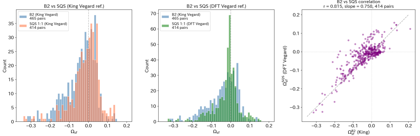
Figure 14: \Omega_{sf} 分布の比較。(左) B2 vs SQS 1:1 (King Vegard 参照)。B2 は負側に偏る。(中) B2 vs SQS 1:1 (DFT Vegard 参照)。DFT 参照でゼロ近傍に集中。(右) B2-SQS 散布図 (DFT Vegard 参照、414 共通ペア)。傾き 0.76。
