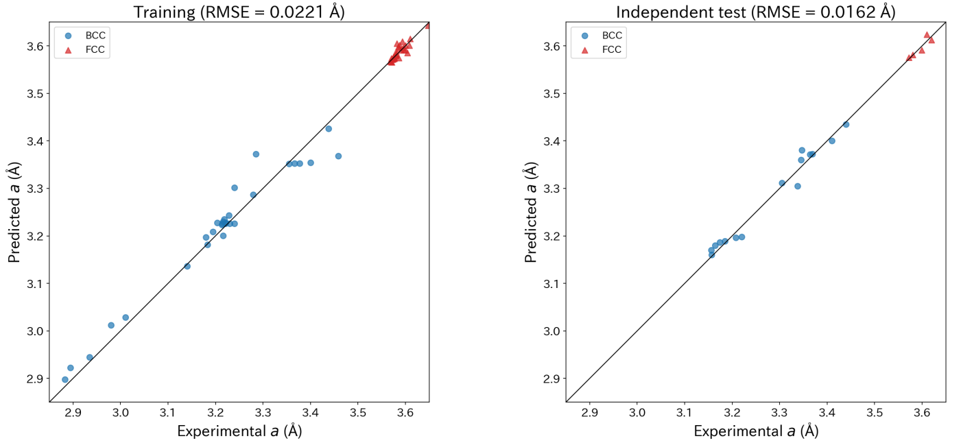
Figure 11: 加法 \delta^{(s)} モデルによる HEA 予測 (64 HEA)。 (a) RMSE 比較。 (b) パリティプロット。 (c) 独立テスト ( q_{BCC} , q_{FCC} は各構造の最適校正定数)。
