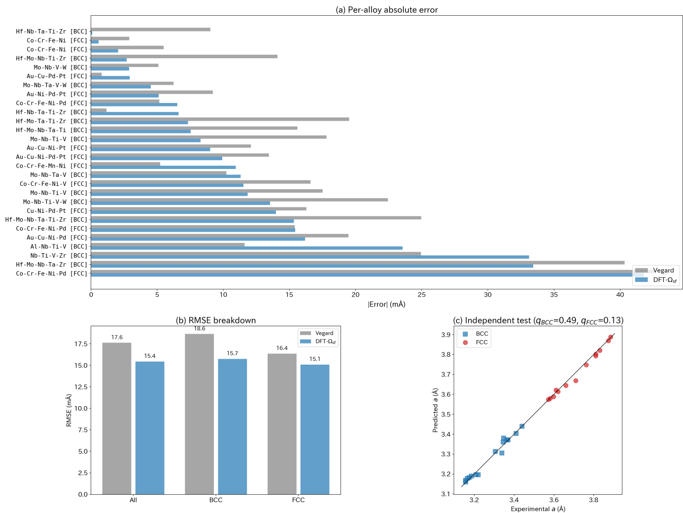
Figure 4: 独立テストセット (28 HEA、12 文献 18 元素) の予測性能。(a) 合金別絶対誤差。(b) 構造別 RMSE (灰: Vegard、青: DFT- \Omega_{\text{sf}} )。 (c) パリティプロット ( q_{\text{BCC}} = 0.49, q_{\text{FCC}} = 0.13 )。BCC 15 合金 (青四角) と FCC 13 合金 (赤丸)。
