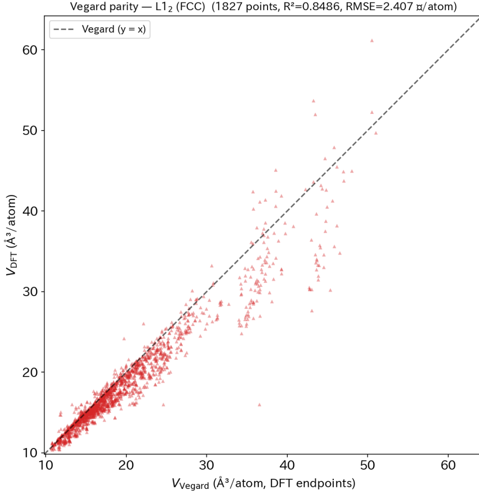
Figure A4: 全 L1_2 ペアの Vegard パリティプロット (1827 点、 R^2 = 0.849 、 RMSE = 2.407 \text{ \AA}^3/\text{atom} )。4f 希土類+Y 除外後は、B2 と同程度の Vegard 則成立精度を示す。
