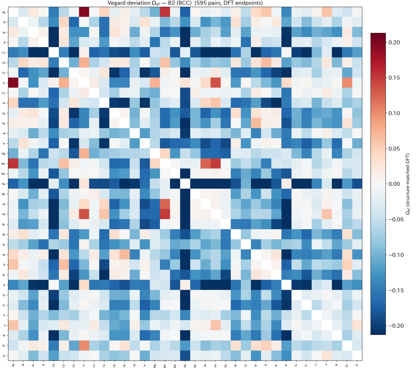
Figure A1: 全元素ペアの B2 (BCC 型) \Omega_{sf} ヒートマップ (595 ペア、35 元素、DFT 端点)。DFT B2 同種体積を端点とした Vegard 偏差。青: 体積収縮 ( \Omega_{sf} < 0 )、赤: 体積膨張 ( \Omega_{sf} > 0 )。大半のペアが負の偏差を示し、B2 秩序構造における体積収縮傾向を反映する。
