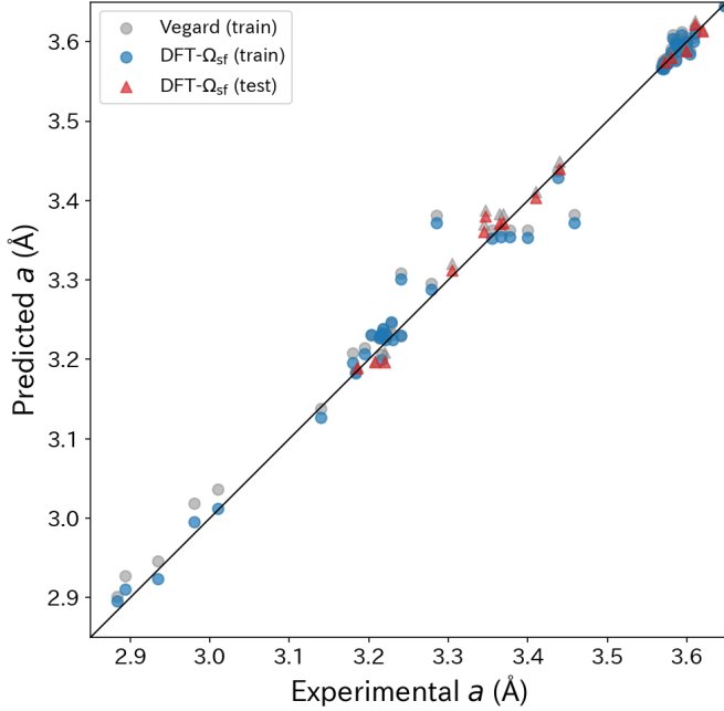
Figure 2: 全 87 HEA のパリティプロット（予測 vs 実験格子定数）。灰色: Vegard 則による予測（64 HEA 訓練セット）、青色: DFT- \Omega_{sf} モデルによる予測（同 64 HEA、RMSE = 0.0214 \text{\AA} ）、赤色三角: 独立テストセット（23 HEA、RMSE = 0.0150 \text{\AA} ）。対角線は a_{\text{pred}} = a_{\text{exp}} を表す。
