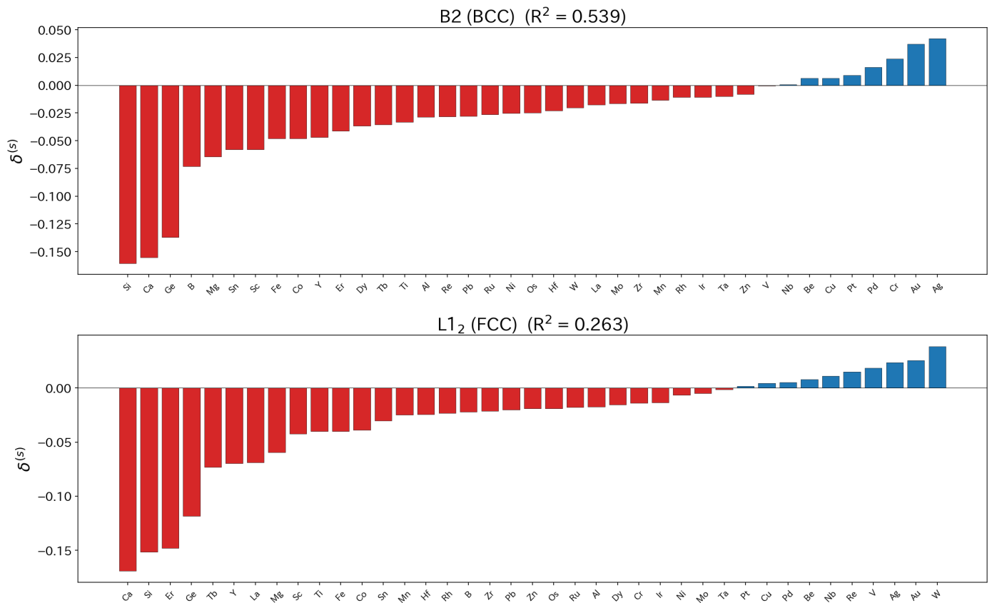
Figure 5: 元素別加法分解パラメータ \delta^{(s)} 。上段: B2 (BCC 参照、 R^2 = 0.54 )、下段: L1 2 (FCC 参照、 R^2 = 0.26 )。赤: 負 (収縮傾向)、青: 正 (膨張傾向)。元素は \delta^{(s)} の昇順にソート。
