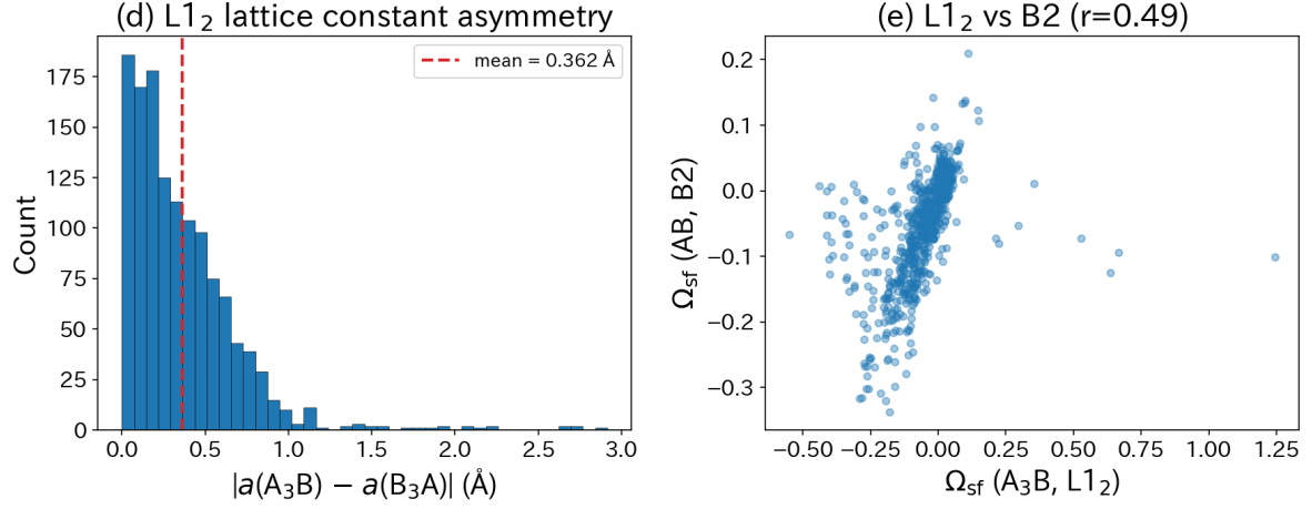
Figure 9: L1 2 構造の非対称性と構造間相関。(d) L1 2 格子定数差 |a(A_3B) - a(B_3A)| の分布 (平均 0.362 Å)。(e) L1 2 \Omega_{sf} vs B2 \Omega_{sf} ( r = 0.49 ) : 構造間で \Omega_{sf} は中程度の相関を持つが一致はしない。
