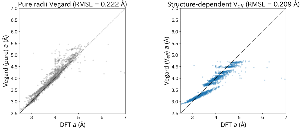
Figure 14: 構造情報吸収による Vegard 則の改善 (全二元系ペア)。左: King 純元素体積による Vegard 予測 (RMSE = 0.222 Å)。右: 構造依存有効体積 V_{\text{eff}} による予測 (RMSE = 0.209 Å)。改善幅は 5.9%にとどまり、二元系レベルでは大部分の分散が組成効果で説明されることを示す。ただし多成分 HEA では 13.4%改善に拡大する (本文参照)。
