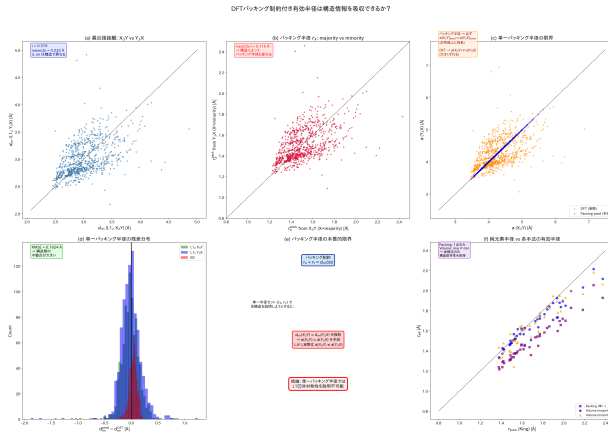
Figure 9: パッキング制約半径の解析。単一半径セットでは a(A_3B) = a(B_3A) を強制するため、L 12 非対称性を表現できない。
