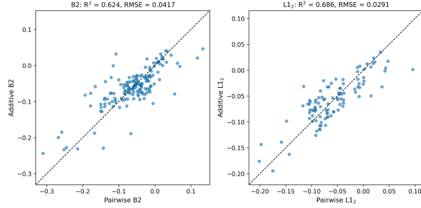
Figure 6: 加法分解のフィット品質。左: B2 ( R^2 = 0.62 )、右: L12 ( R^2 = 0.69 )。横軸: ペアワイズ \Omega_{sf} 、縦軸: 加法モデル予測 \delta_A + \delta_B 。破線は完全一致。
