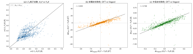
Figure 10: L 12 格子定数の非対称性。 a(A_3B) - a(B_3A) の分布は対称だが大きな分散を持つ。
