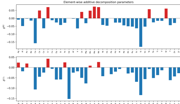
Figure 5: 元素別加法分解パラメータ \delta 。上: B2 、下: L1_2 。赤: 正 (格子膨張)、青: 負 (格子収縮)。
