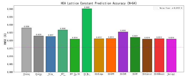
Figure 2: 各手法の RMSE 比較棒グラフ。破線はノイズフロア \sigma \approx 0.016 Å を示す。
