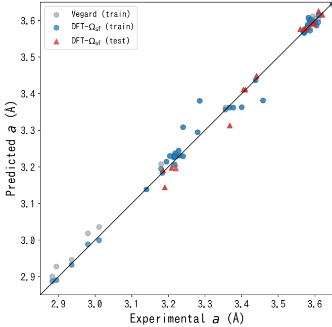
Figure 1: パリティプロット (予測 vs 実験格子定数)。灰丸: Vegard 則 (64 HEA)、青丸: DFT- \Omega_{sf} (64 HEA, RMSE = 0.0214 Å)、赤三角: 独立テスト (23 HEA)。FCC RMSE = 0.0133 Å (Vegard 比 18.9%改善)。実線は完全一致線。
