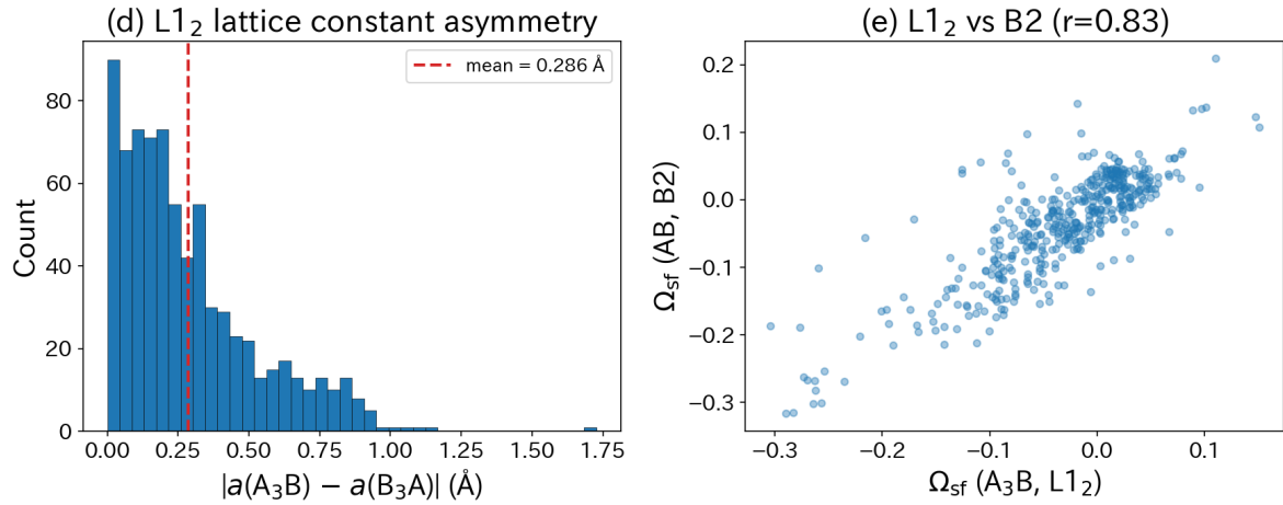
Figure A8: L_{12} 構造の非対称性と構造間相関。(d) L_{12} 格子定数差 |a(A_3B) - a(B_3A)| の分布 (754 ペア、平均 0.286 \text{ \AA} )。 (e) L_{12} \Omega_{sf} vs B_2 \Omega_{sf} (435 ペア、 r = 0.83 ) : 構造間で \Omega_{sf} は強い相関を持つが完全には一致しない。
