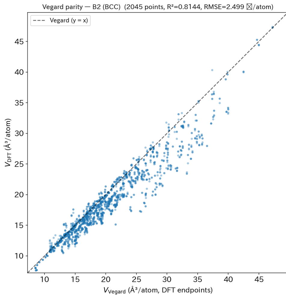
Figure H.20: 全 B2 ペアの Vegard パリティプロット (2045 点、 R^2 = 0.81 、RMSE = 2.50 Å 3 /atom)。横軸: 構造整合 DFT 端点による Vegard 予測体積、縦軸: DFT 計算体積。破線は y = x (Vegard 完全成立)。
