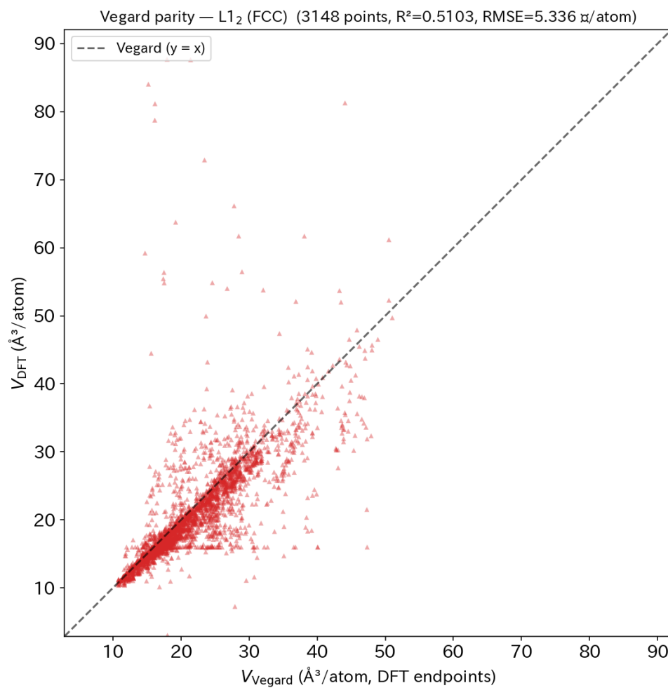
Figure H.21: 全 L1 2 ペアの Vegard パリティプロット (3148 点、 R^2 = 0.51 、RMSE = 5.34 Å 3 /atom)。B2 に比べ散乱が大きく、4f 希土類の異常点が上方に突出する。
