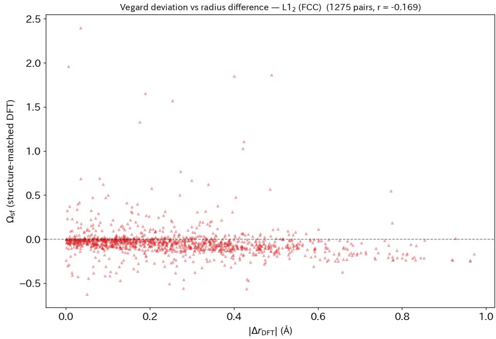
Figure H.23: L1 2 \Omega_{sf} と純元素 DFT 半径差の関係 (1275 ペア、 r = -0.17 )。B2 に比べ相関が弱く、 \Omega_{sf} はサイズ差だけでは説明できない。
