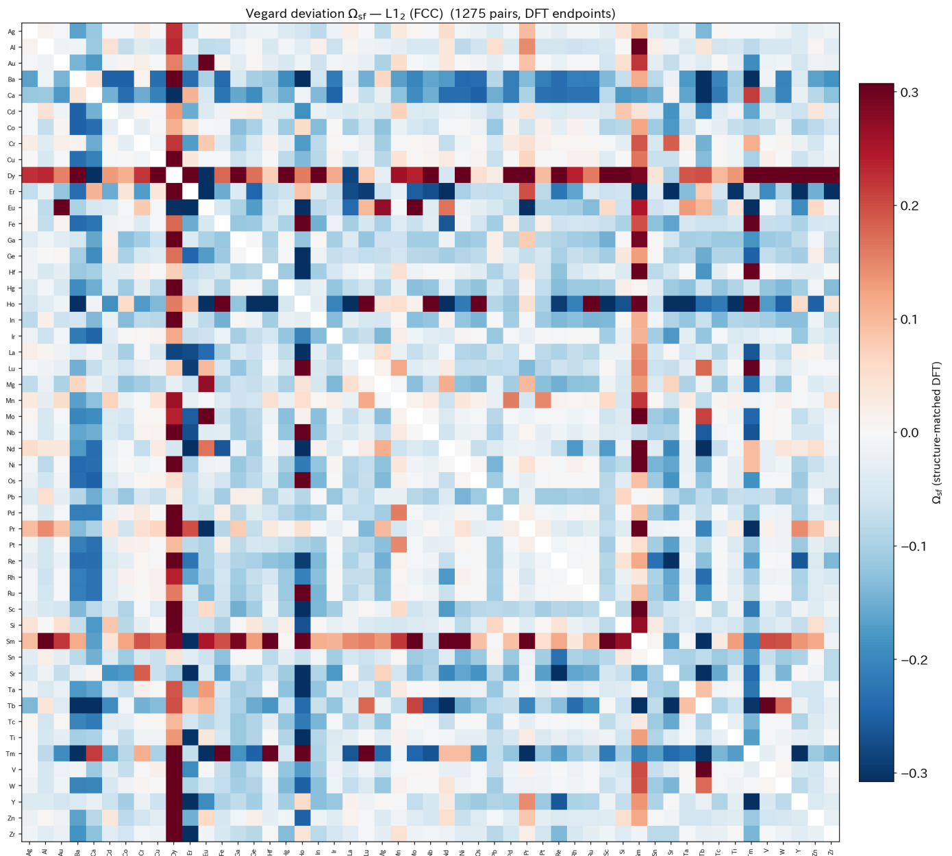
Figure H.19: 全元素ペアの L1_2 (FCC 型) \Omega_{sf} ヒートマップ (1275 ペア、51 元素)。DFT L1_2 同種体積を端点とした Vegard 偏差。Dy, Er, Tb, Sm 等の希土類 4f 元素が行・列で極端な正の偏差を示す。
