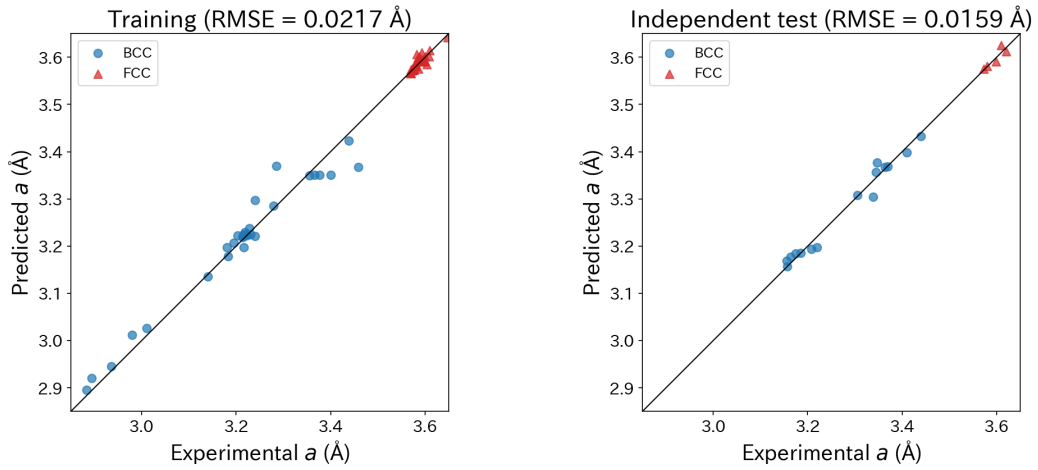
Figure 13: 加法 \delta^{(s)} モデルによる HEA 予測 (64 HEA)。 (a) RMSE 比較。 (b) パリティプロット。 (c) 独立テスト ( q_{\text{BCC}} , q_{\text{FCC}} は各構造の最適校正定数)。
