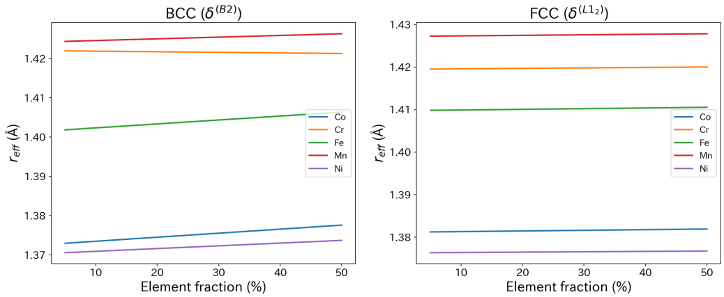
Figure 14: 組成依存有効半径 r_{\text{eff}} 。 CoCrFeMnNi 系 FCC 合金における各元素の r_{\text{eff}} の組成依存性。
