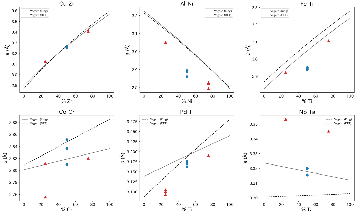
Figure 7: 代表6元素ペアの組成軸 Vegard プロット。破線: King 原子体積 (実験値) から算出した Vegard 則 (B2 換算)、実線: DFT 純元素体積から算出した Vegard 則 (GGA 系統誤差を含む)、青丸: DFT B2 計算値 ( c = 50\% )、赤三角: DFT L1_2 計算値 ( c = 25\%, 75\% 、B2 等価スケールに変換)。DFT 点と実線の乖離が \Omega_{sf} の構造依存成分に対応する。
