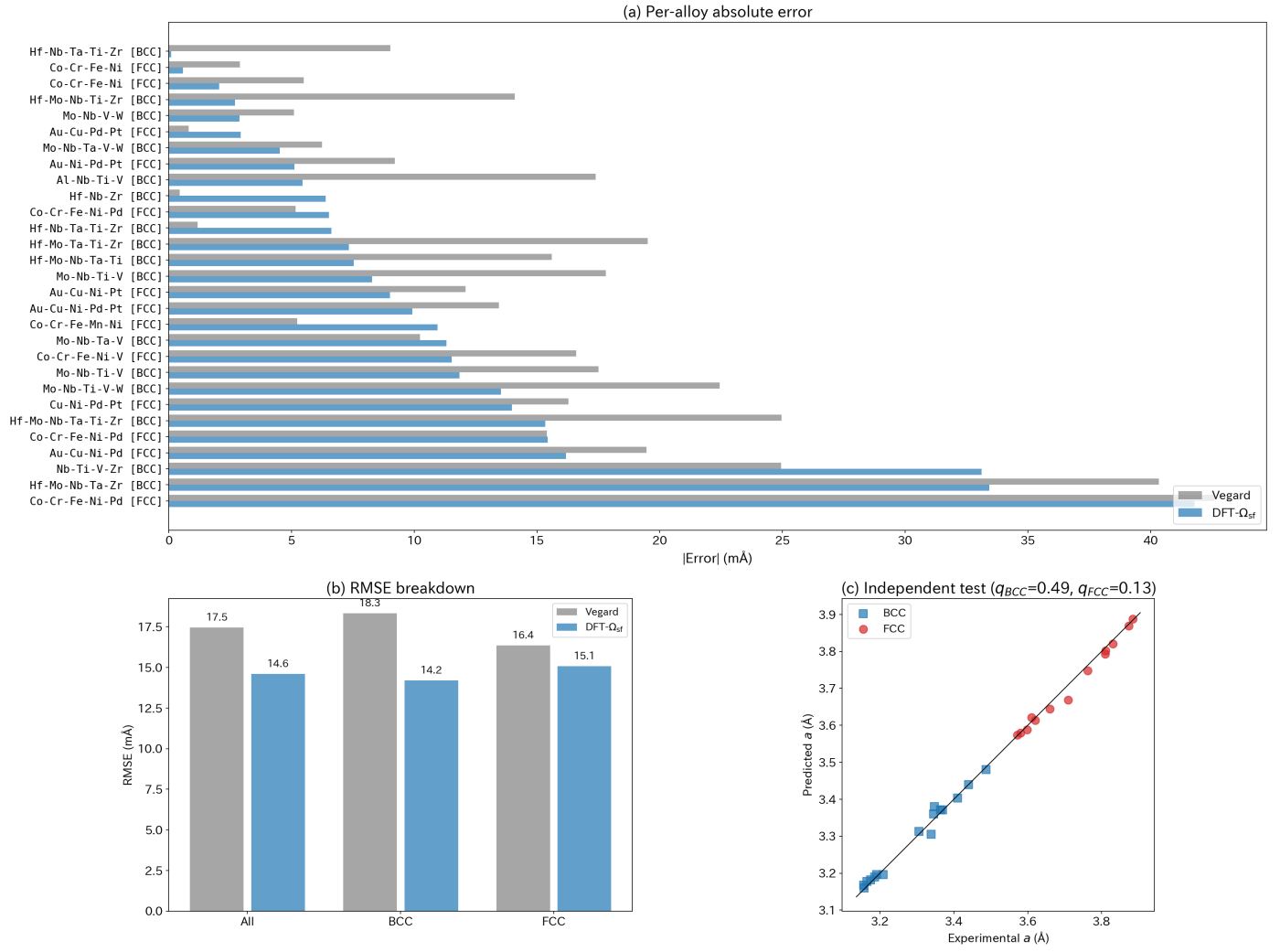
Figure 4: 独立テストセット (29 HEA、13 文献 19 元素) の予測性能。(a) 合金別絶対誤差。(b) 構造別 RMSE (灰: Vegard、青: DFT- \Omega_{sf} )。 (c) パリティプロット ( q_{BCC}=0.49, q_{FCC}=0.13 )。BCC 16 合金 (青四角) と FCC 13 合金 (赤丸)。
