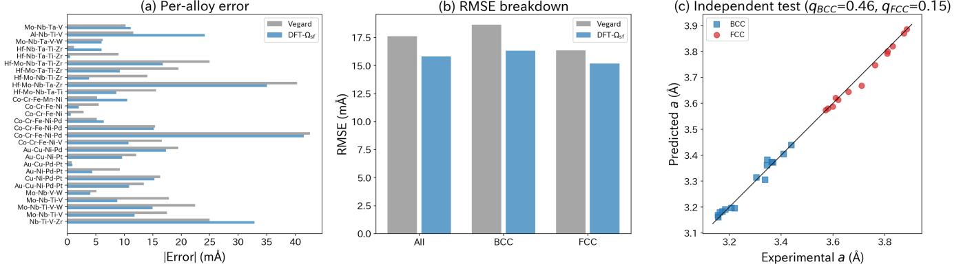
Figure 4: 独立テストセット (28 HEA、12 文献 18 元素) の予測性能。(a) 合金別絶対誤差。(b) 構造別 RMSE (灰: Vegard、青: DFT- \Omega_{sf} )。 (c) パリティプロット ( q_{BCC} = 0.46 , q_{FCC} = 0.15 )。BCC 15 合金 (青四角) と FCC 13 合金 (赤丸)。
