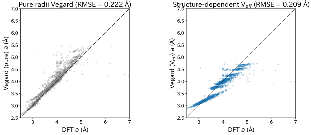
Figure 14: 構造情報吸収による Vegard 則の改善 (全二元系ペア)。左: King 純元素体積による Vegard 予測 (RMSE = 0.222 Å)。右: 構造依存有効体積 V_{\text{eff}} による予測 (RMSE = 0.209 Å)。改善幅は 5.9%にとどまり、二元系レベルでは大部分の分散が組成効果で説明されることを示す。
