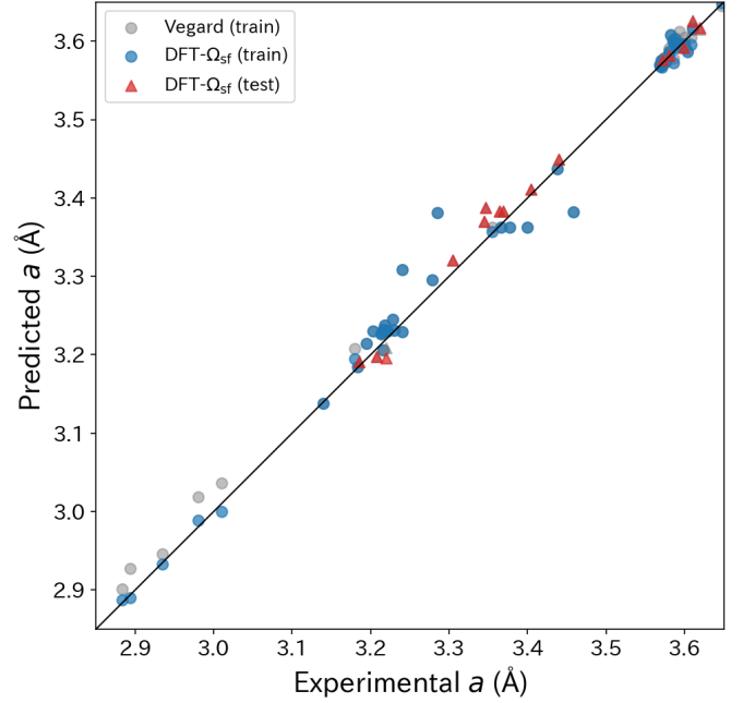
Figure 2: パリティプロット (予測 vs 実験格子定数)。灰丸: Vegard 則 (64 HEA)、青丸: DFT- \Omega_{sf} (64 HEA、RMSE = 0.0214 Å)、赤三角: 独立テスト (23 HEA)。独立テスト全体 RMSE = 0.0150 Å (Vegard 比 13.4%改善)。実線は完全一致線。
