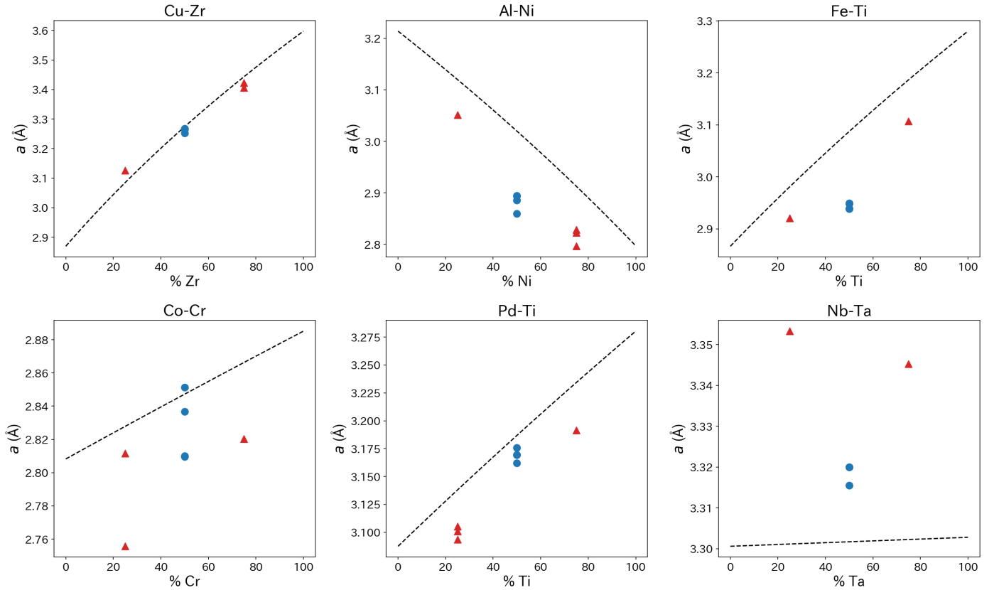
Figure 8: 代表 6 元素ペアの組成軸 Vegard プロット。破線: Vegard 則、丸印: DFT 計算値 (L1 2 B 3 A, B2 AB, L1 2 A 3 B)。
