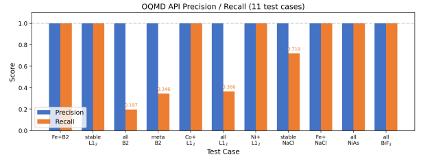
Figure 4: OQMD API 正解データに対する Precision (青) と Recall (橙)。全 11 テストで Precision = 1.0 を達成。A04/A05/A10/N01 の低 Recall はデータ不正確性ではなく LIMIT 100 制約による。C08 (API フィルタ非対応) は比較対象外として除外した。
