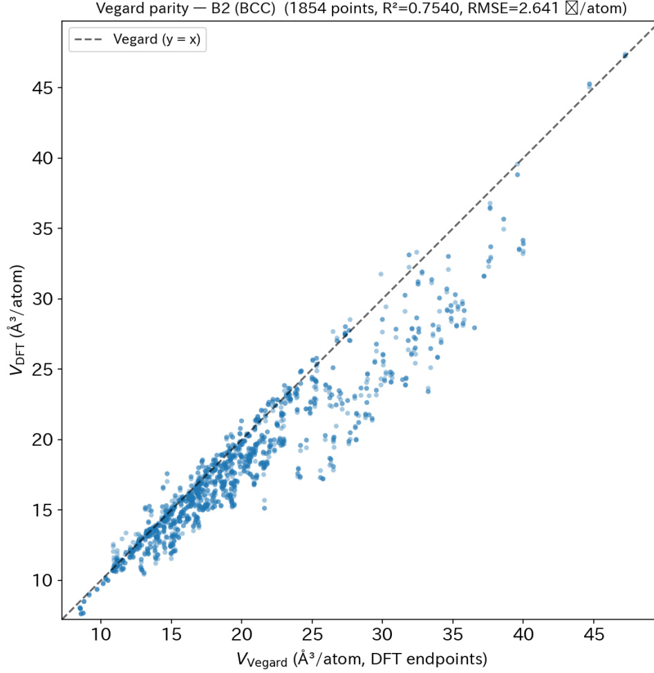
Figure A3: 全 B2 ペアの Vegard パリティプロット (1854 点、 R^2 = 0.754 、 RMSE = 2.641 \text{ \AA}^3/\text{atom} )。横軸: 構造整合 DFT 端点による Vegard 予測体積、縦軸: DFT 計算体積。破線は y = x (Vegard 完全成立)。
