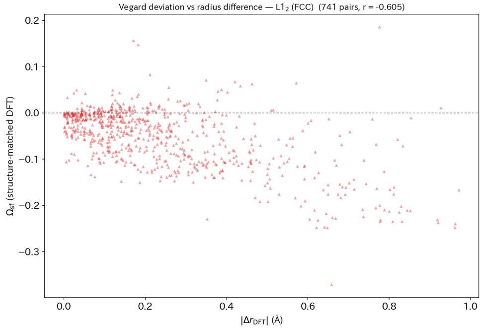
Figure A6: L1 2 \Omega_{sf} と純元素 DFT 半径差の関係 (741 ペア、 r = -0.61 )。B2 よりも強い負の相関を示し、サイズ差が大きいかほど体積収縮が増大する。
