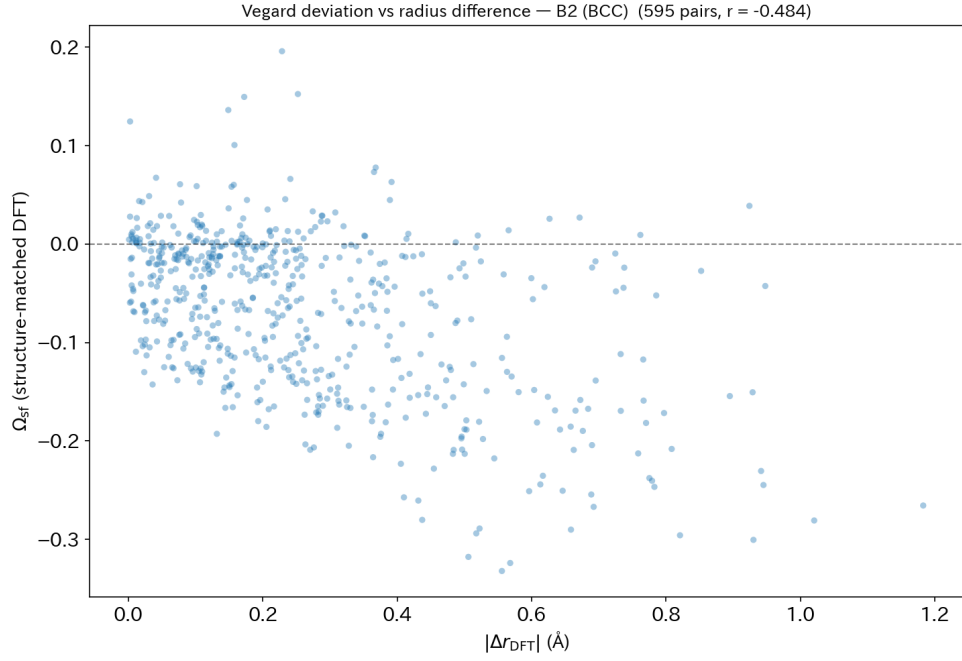
Figure A5: B2 \Omega_{sf} と純元素 DFT 半径差の関係 (595 ペア、 r = -0.48 )。半径差が大きいかほど体積収縮（負の \Omega_{sf} ）が増大する傾向。
