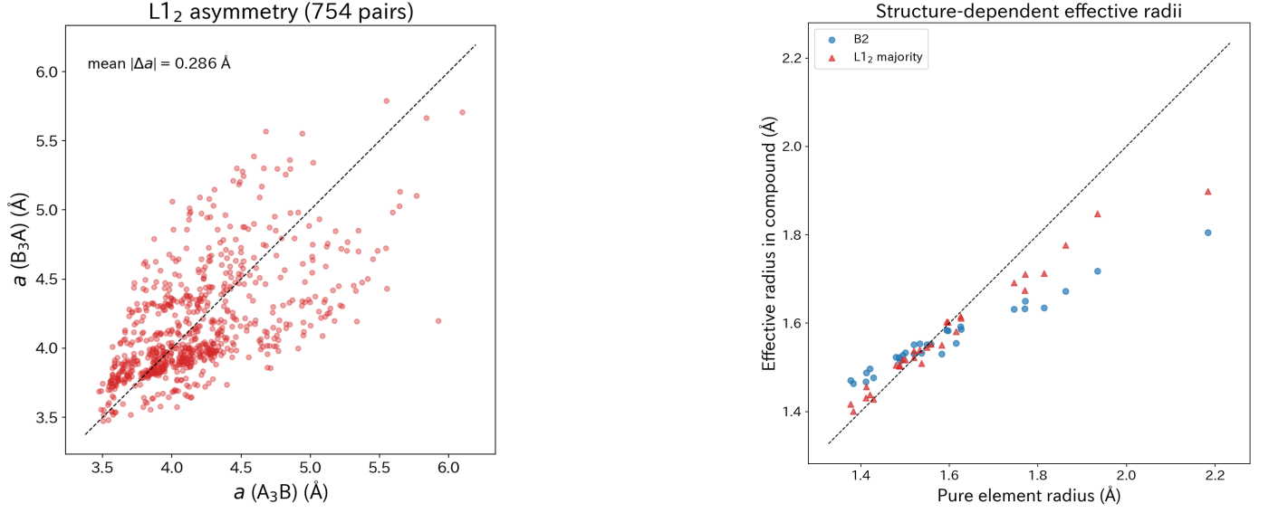
Figure 12: (左) L1 2 格子定数非対称性 |a(A_3B) - a(B_3A)| (754 ペア、平均 = 0.286 Å、std = 0.24 Å)。 (右) 構造依存有効半径。少数派サイトの偏差が多数派より 179%大きい。
