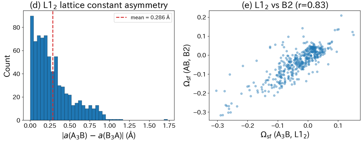
Figure 10: L1_2 構造の非対称性と構造間相関。(d) L1_2 格子定数差 |a(A_3B) - a(B_3A)| の分布 (754 ペア、平均 0.286 Å)。(e) L1_2 \Omega_{sf} vs B2 \Omega_{sf} (435 ペア、 r = 0.83 ) : 構造間で \Omega_{sf} は強い相関を持つが完全には一致しない。
