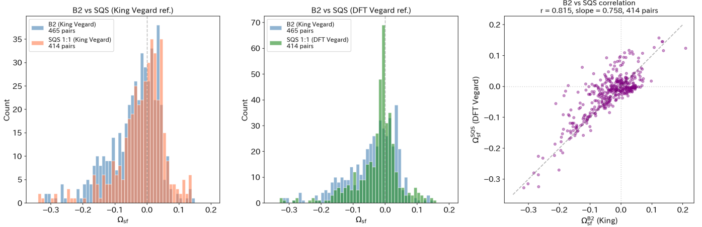
Figure 18: \Omega_{sf} 分布の比較。(左) B2 vs SQS 1:1 (King Vegard 参照)。B2 は負側に偏る。(中) B2 vs SQS 1:1 (DFT Vegard 参照)。DFT 参照でゼロ近傍に集中。(右) B2–SQS 散布図 (DFT Vegard 参照、414 共通ペア)。傾き 0.76。
