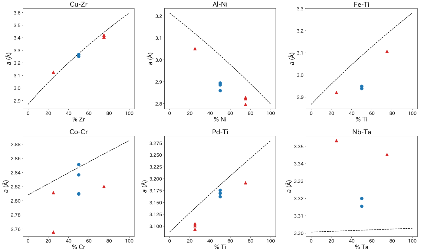
Figure 7: 代表 6 元素ペアの組成軸 Vegard プロット。横軸：元素 B の原子分率 c_B ( 0 \rightarrow 1 )、縦軸：格子定数 ( \text{\AA} )。破線：Vegard 則の線形補間 (純元素体積から)。丸印：DFT 計算値 ( B_3A at c_B = 0.25 , AB ( B_2 ) at c_B = 0.50 , A_3B at c_B = 0.75 )。各点の数値は \Omega_{\text{sf}} 値。同一ペアでも L_{12} A_3B と B_3A で偏差方向・大きさが異なり、3 構造の DFT 点は Vegard 線上にも滑らかな曲線上にも乗らない。これは \Omega_{\text{sf}} が組成比だけでなく構造 (配位環境) に依存することの直接的証拠である。
