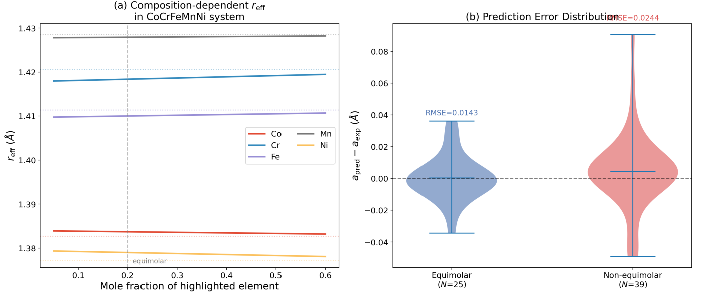
Figure 13: 組成依存有効半径。(a) CoCrFeMnNi 系 FCC 合金における各元素の r_{\text{eff}} の組成依存性 (1 成分を変化、残りは均等配分)。破線は純元素半径。(b) 等モル vs 非等モル HEA の予測誤差分布。
