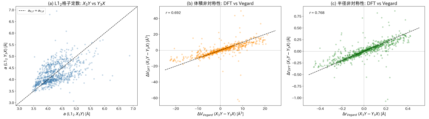
Figure 10: L1 2 格子定数の非対称性。 a(A_3B) - a(B_3A) の分布は対称だが大きな分散を持つ。
