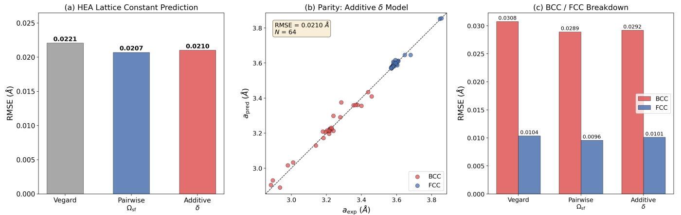
Figure 12: 加法分解 \delta^{(s)} モデルによる HEA 格子定数予測。(a) 3 手法の RMSE 比較。(b) パリティプロット（予測 vs 実験）。(c) BCC/FCC 構造別 RMSE 分解。
