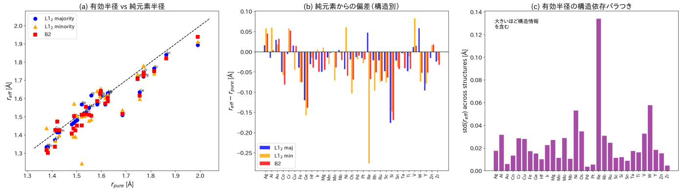
Figure 11: 構造依存有効半径。多数派サイト（面心）と少数派サイト（頂点）で異なる有効半径を持つ。純元素半径からの偏差は少数派サイトのほうが大きい。
