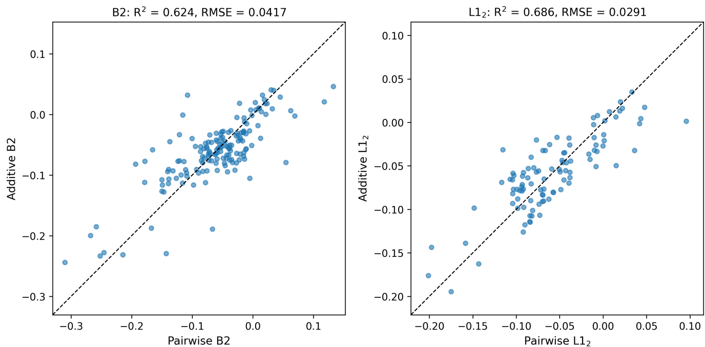
Figure 6: 加法分解のフィット品質。左: B2 ( R^2 = 0.62 )、右: L1 2 ( R^2 = 0.69 )。横軸: ペアワイズ \Omega_{sf}^{(s)} 、縦軸: 加法モデル予測 \delta_A^{(s)} + \delta_B^{(s)} 。破線は完全一致。
