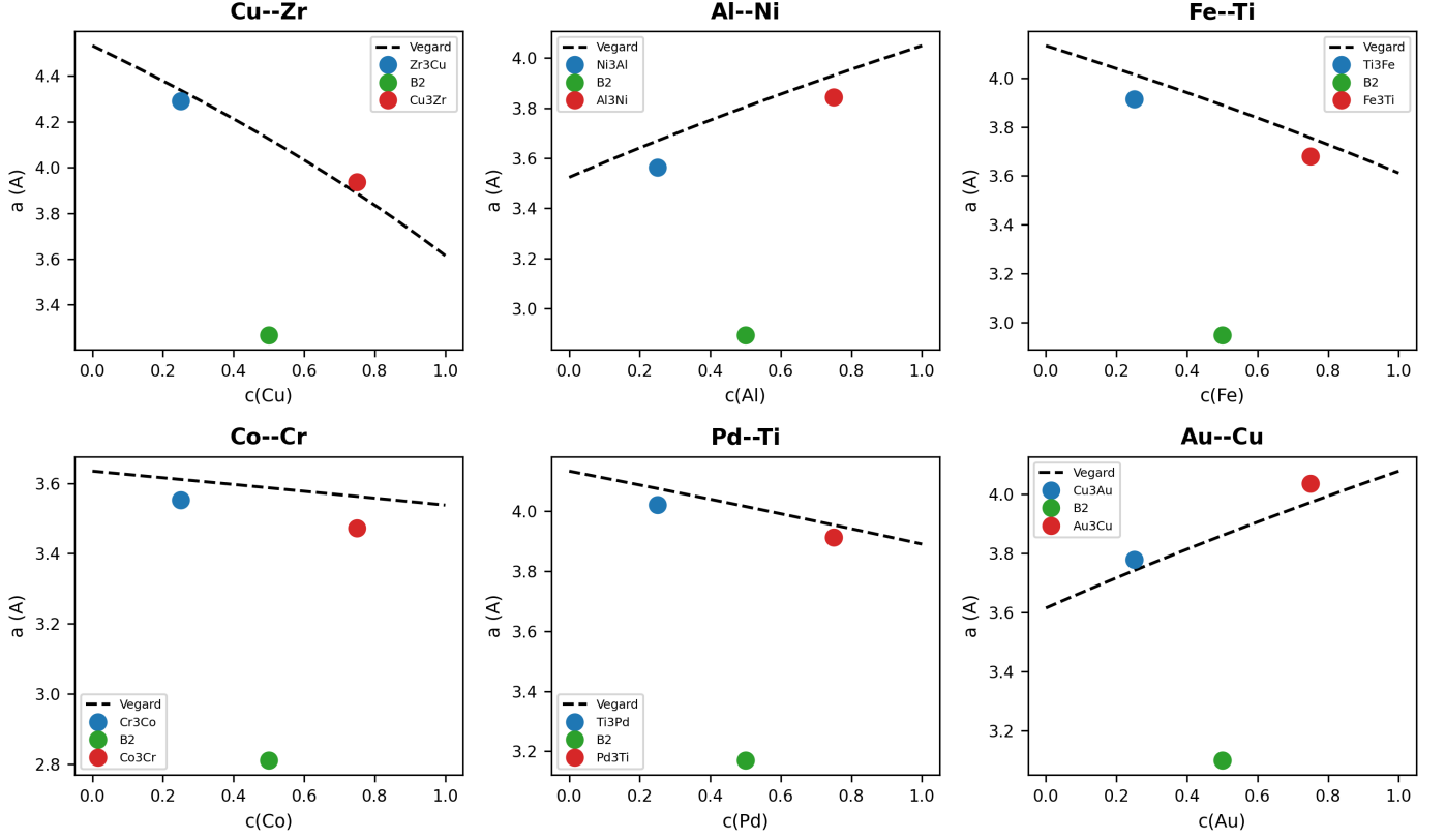
Figure 7: 代表 6 ペアの組成軸 Vegard プロット。破線：Vegard 則の線形補間。丸：DFT 計算による格子定数。Vegard 則からの偏差 ( \Omega_{sf} ) が元素ペアにより正・負両方に現れ、かつ組成比 ( A_3B vs B_3A ) で大きく異なることが可視化される。
