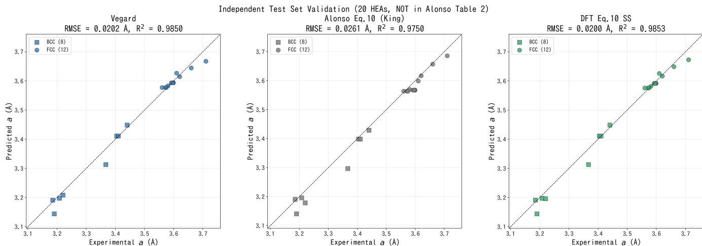
Figure 4: 独立テストセット (20 HEA) の予測精度。縦軸：予測格子定数、横軸：実験格子定数。
