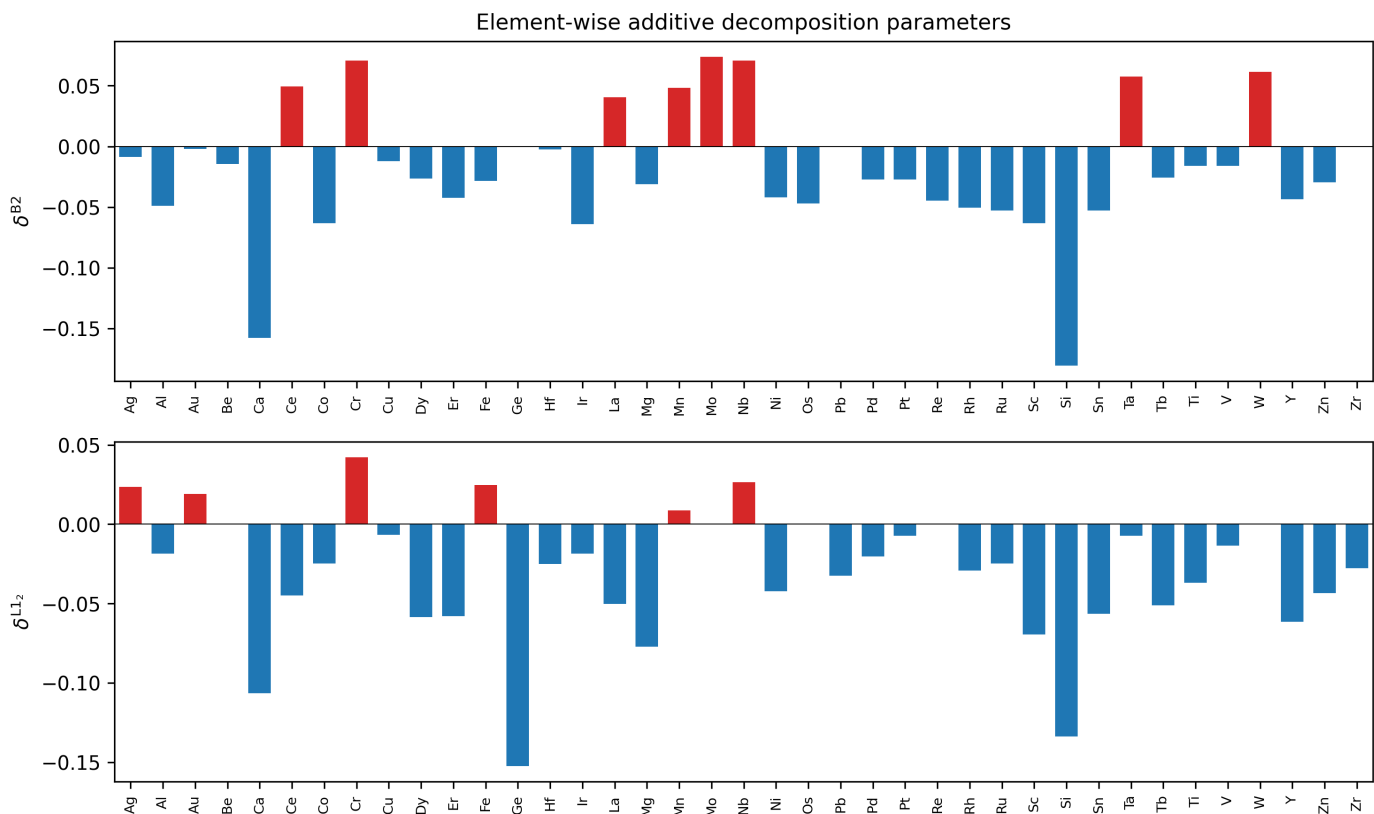
Figure 5: 元素別加法分解パラメータ \delta 。上: B2、下: L1 2 。赤: 正 (格子膨張)、青: 負 (格子収縮)。
