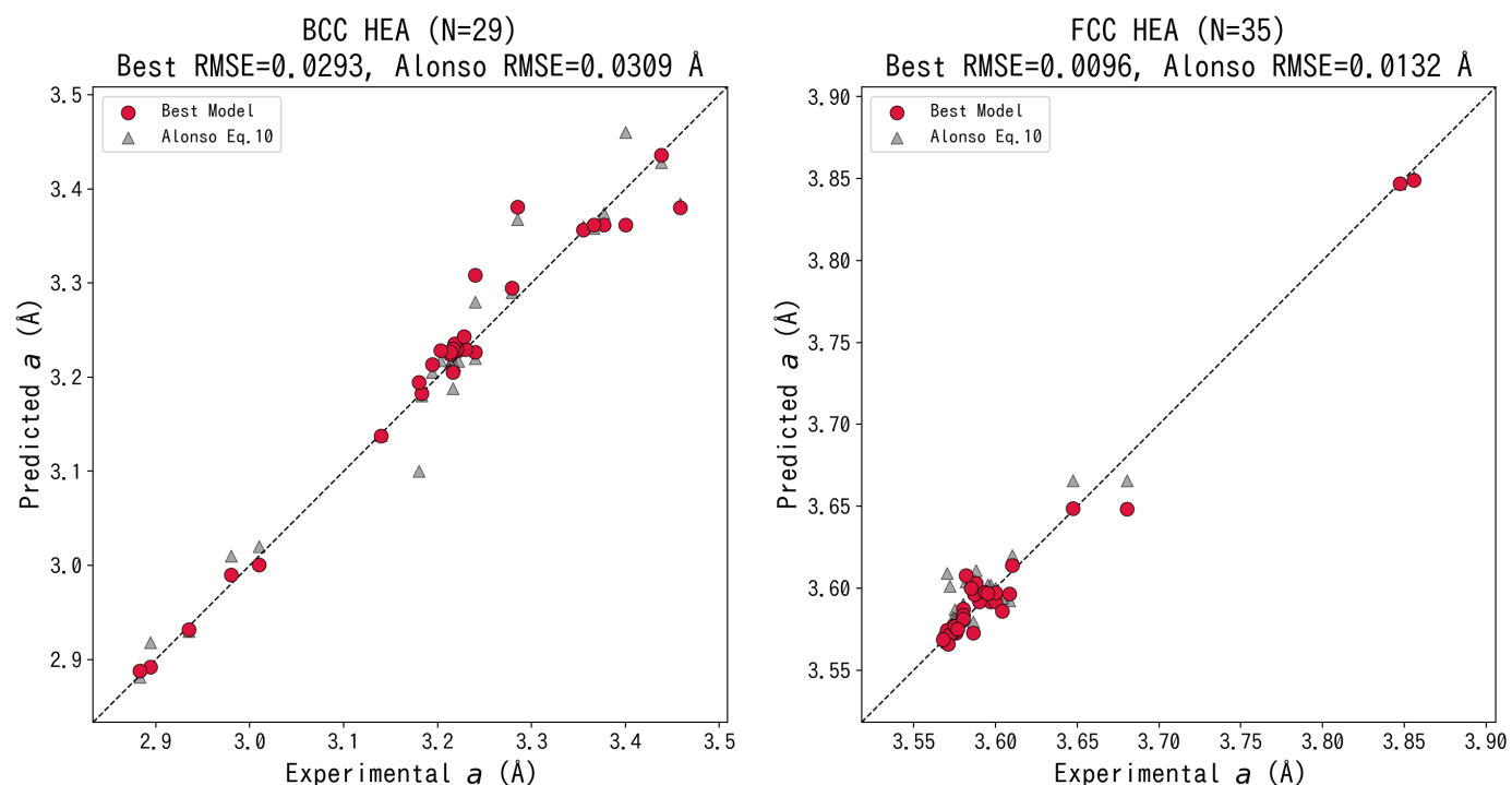
Figure 3: BCC (左) と FCC (右) 別のパリティプロット。FCC HEA は対角線に極めて近い。
