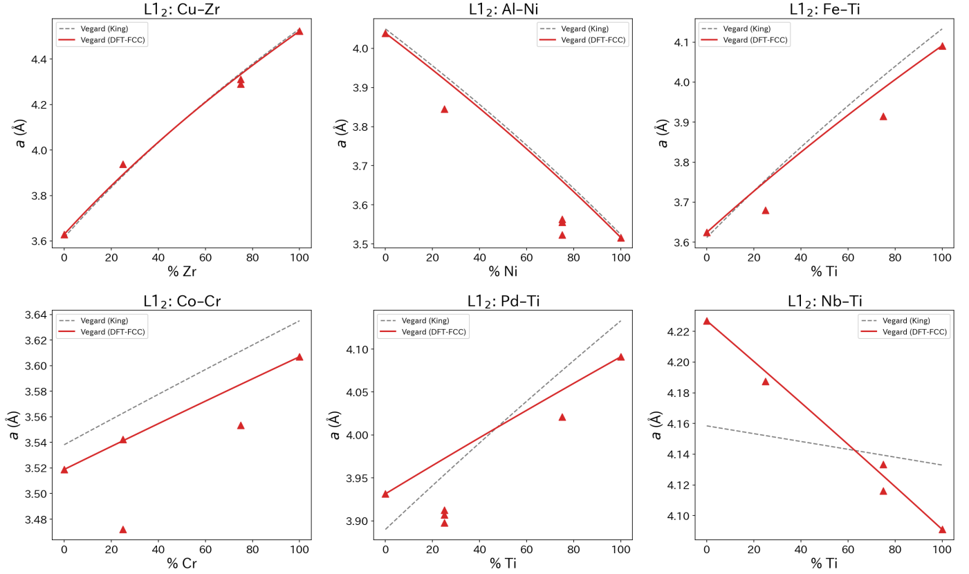
Figure 8: 代表 6 元素ペアの L1_2 (FCC 型) Vegard プロット。破線: King 原子体積 (実験値) から算出した Vegard 則、実線: DFT L1_2 同種体積 V_X^{\text{FCC}} = a_{L1_2}(X-X)^3/4 を端点とした Vegard 則。赤三角: DFT L1_2 計算値 ( c = 0, 25, 75, 100\% )。構造整合の端点を用いることで、BCC/FCC 間の構造体積差アーティファクトを排除し、 \Omega_{\text{sf}} をクリーンに評価できる。
