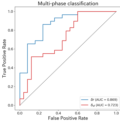
Figure 16: SS vs 非 SS 分類の ROC 曲線 (54 HEA)。 \delta r (AUC = 0.869) が \delta_{\text{sf}} (AUC = 0.723) を上回る。
