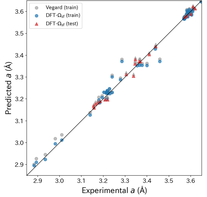
Figure 2: 全 87 HEA のパリティプロット (予測 vs 実験格子定数)。灰色: Vegard 則による予測 (64 HEA 訓練セット)、青色: DFT- \Omega_{sf} モデルによる予測 (同 64 HEA、RMSE = 0.0214 Å)、赤色三角: 独立テストセット (28 HEA、RMSE = 0.0154 Å)。対角線は a_{pred} = a_{exp} を表す。
