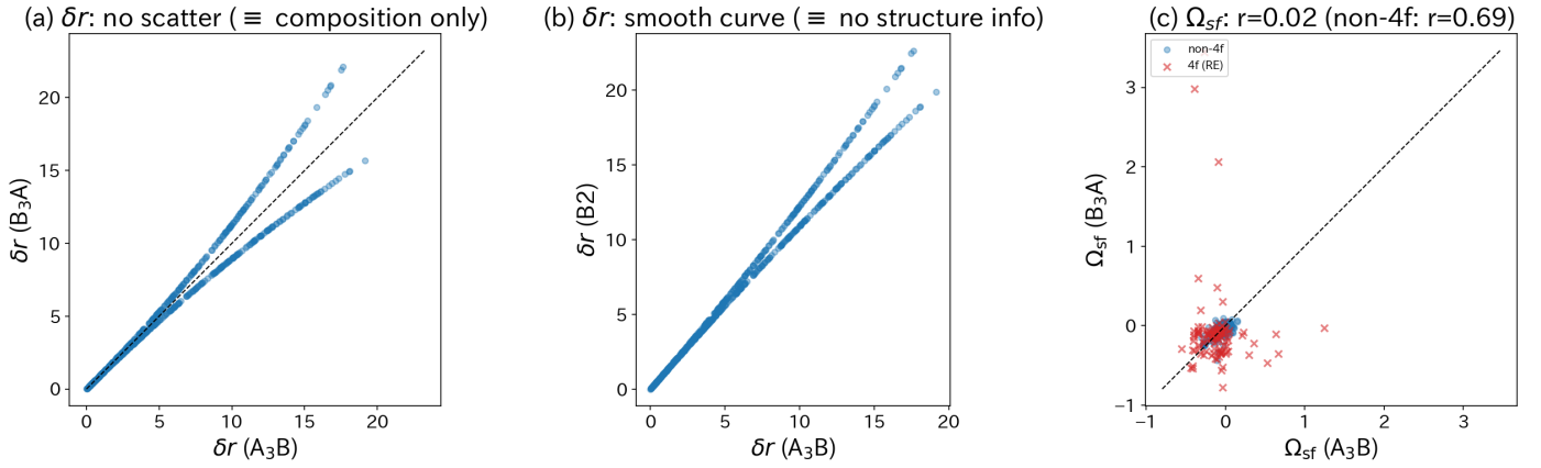
Figure 9: \delta r の構造不変性の証明 (595 ペア)。(a) \delta r(A_3B) vs \delta r(B_3A) : 完全一致 (構造情報ゼロ)。(b) \delta r(A_3B) vs \delta r(B_2) : 滑らかな曲線 (組成のみの関数)。(c) \Omega_{\text{sf}}(A_3B) vs \Omega_{\text{sf}}(B_3A) : 全体 r = 0.02 (青丸: 非 4f 465 ペア r = 0.69 、赤 \times : 4f 希土類 130 ペア)。4f 元素の GGA 過大評価が低相関の主因。
