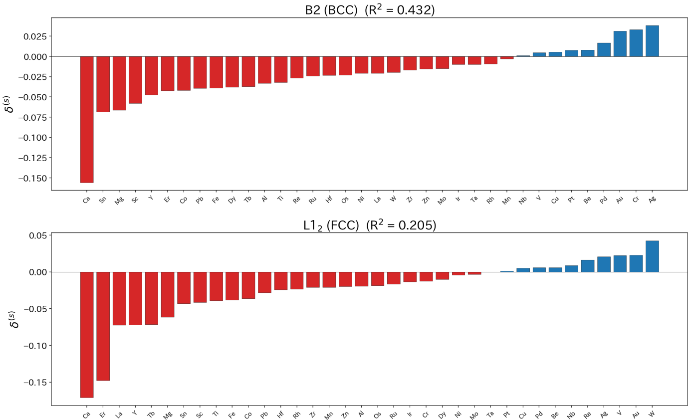
Figure 5: 元素別加法分解パラメータ \delta^{(s)} 。上段: B2 (BCC 参照, R^2 = 0.43 )、下段: L1_2 (FCC 参照, R^2 = 0.20 )。赤: 負 (収縮傾向)、青: 正 (膨張傾向)。元素は \delta^{(s)} の昇順にソート。
