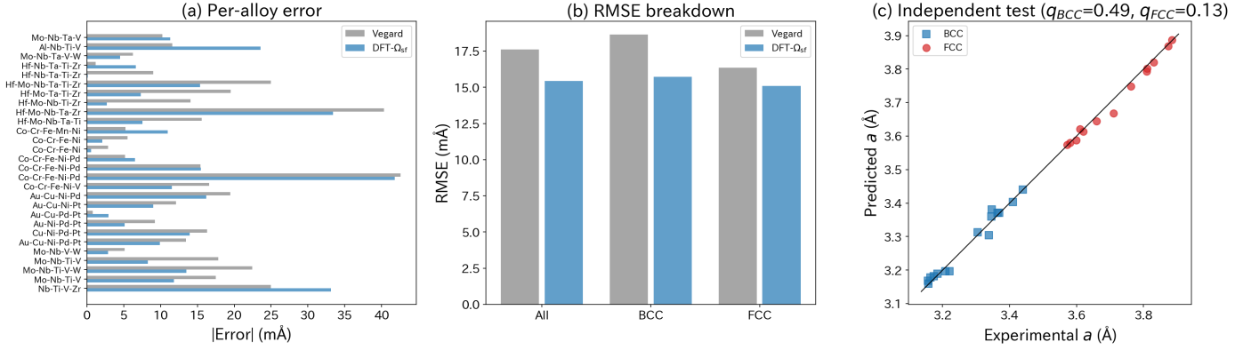
Figure 4: 独立テストセット (28 HEA、12 文献 18 元素) の予測性能。(a) 合金別絶対誤差。(b) 構造別 RMSE (灰: Vegard、青: DFT- \Omega_{sf} )。 (c) パリティプロット ( q_{BCC}=0.49 , q_{FCC}=0.13 )。BCC 15 合金 (青四角) と FCC 13 合金 (赤丸)。
