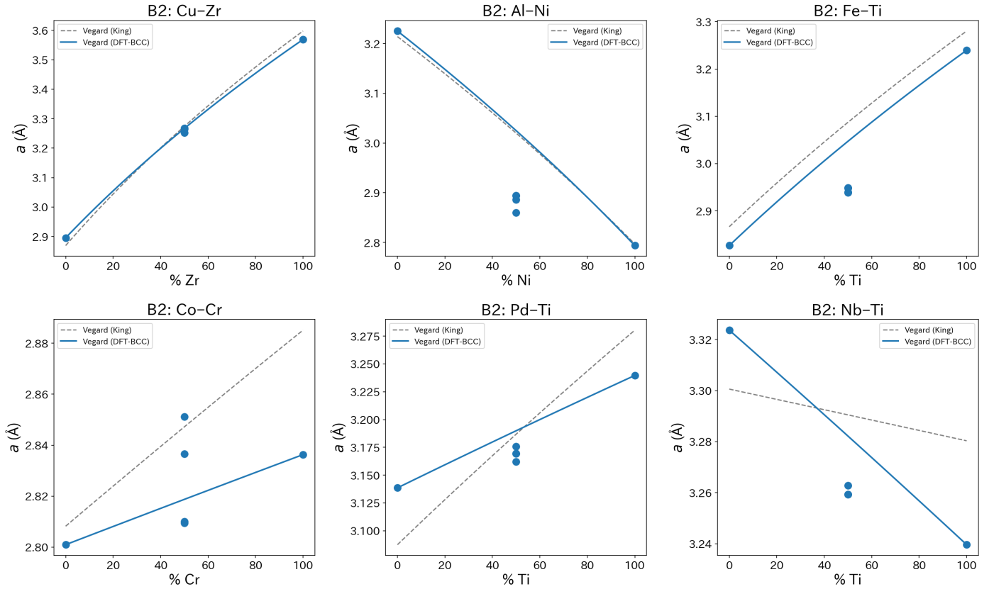
Figure 7: 代表 6 元素ペアの B2 (BCC 型) Vegard プロット。破線: King 原子体積 (実験値) から算出した Vegard 則、実線: DFT B2 同種体積 V_X^{BCC} = a_{B2}(X-X)^3/2 を端点とした Vegard 則。青丸: DFT B2 計算値 ( c = 0, 50, 100\% )。DFT 同種端点を基準とすることで、GGA 系統誤差が相殺され、点と実線の偏差が純粋な \Omega_{sf} に対応する。
