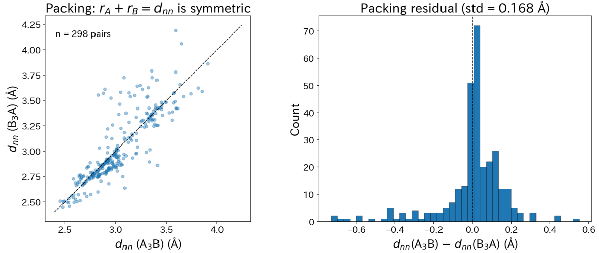
Figure 9: 剛体球接触モデル半径の解析。剛体球モデル ( d_{nn} = r_A + r_B ) で推定した半径による格子定数予測と実際の DFT 格子定数の比較。単一半径セットでは r_A + r_B が対称操作であるため a(A_3B) = a(B_3A) を強制し、 L1_2 の非対称性（平均差 0.328 Å）を表現できない。結果として RMSE = 0.162 Å と Vegard 則の 5 倍以上の残差が生じる。
