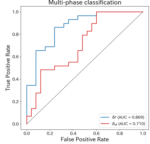
Figure 16: SS vs 非 SS 分類の ROC 曲線 (54 HEA)。 \delta r (AUC = 0.869) が \delta_{\text{sf}} (AUC = 0.710) を上回る。
