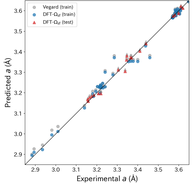
Figure 2: 全 87 HEA のパリティプロット (予測 vs 実験格子定数)。灰色: Vegard 則による予測 (64 HEA 訓練セット)、青色: DFT- \Omega_{sf} モデルによる予測 (同 64 HEA、RMSE = 0.0214 Å)、赤色三角: 独立テストセット (28 HEA、RMSE = 0.0154 Å)。対角線は a_{\text{pred}} = a_{\text{exp}} を表す。
