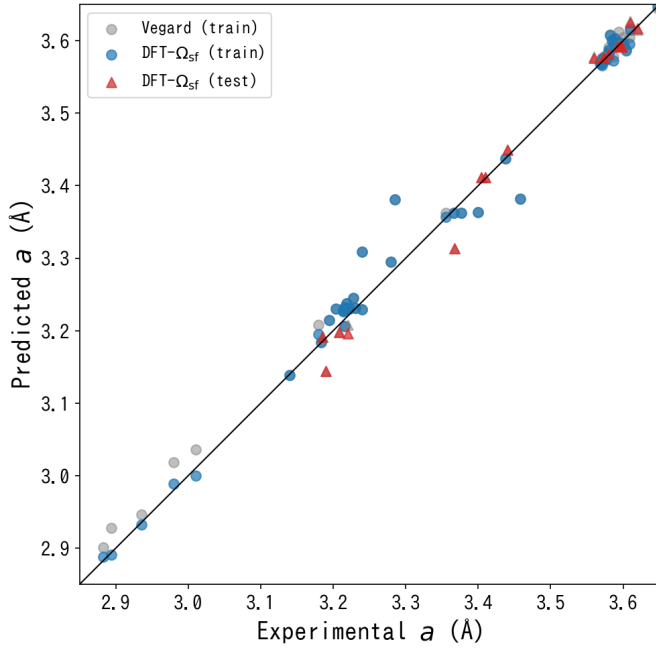
Figure 1: B2/L1 2 参照 DFT- \Omega_{sf} モデルのパリティプロット (予測格子定数 vs 実験格子定数)。灰丸: Vegard 則 (訓練 64 HEA)、青丸: DFT- \Omega_{sf} (B2/L1 2 参照、訓練 64 HEA、RMSE = 0.0214 Å)、赤三角: DFT- \Omega_{sf} (B2/L1 2 参照、独立テスト 20 HEA、RMSE = 0.0222 Å)。実線は完全一致線 ( a_{pred} = a_{exp} )。DFT- \Omega_{sf} モデルは Vegard 則に比べ系統的に対角線に近いが、BCC HEA ( a > 3.1 Å) では独立テストで偏差が残る。これは B2 秩序構造 ( \alpha = -1 ) の \Omega_{sf} がランダム固溶体の体積偏差を大きく評価してしまうためであり、SQS 参照への変更で改善される (4.12 節)。
