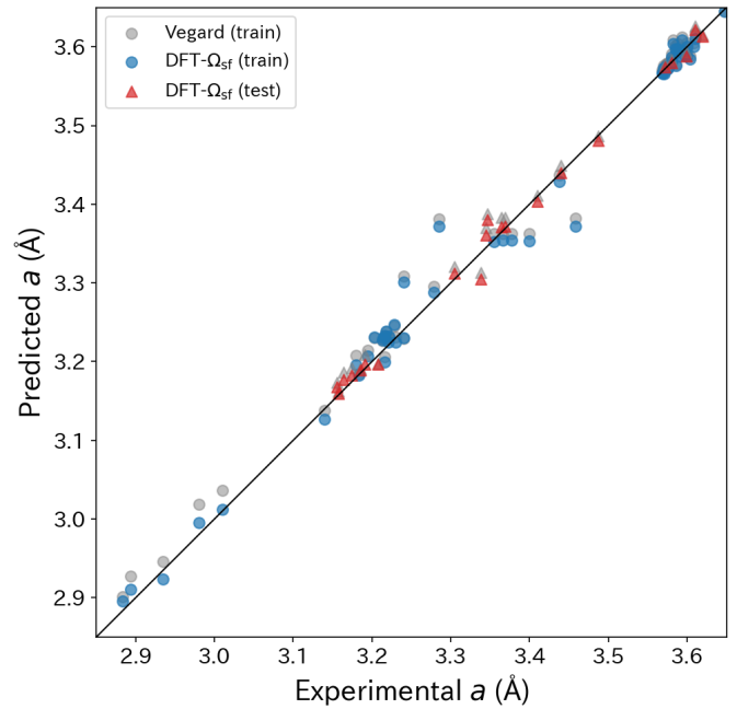
Figure 2: 全 87 HEA のパリティプロット (予測 vs 実験格子定数)。灰色: Vegard 則による予測 (64 HEA 訓練セット)、青色: DFT- \Omega_{\text{sf}} モデルによる予測 (同 64 HEA、RMSE = 0.0214 Å)、赤色三角: 独立テストセット (29 HEA、RMSE = 0.0146 Å)。対角線は a_{\text{pred}} = a_{\text{exp}} を表す。
