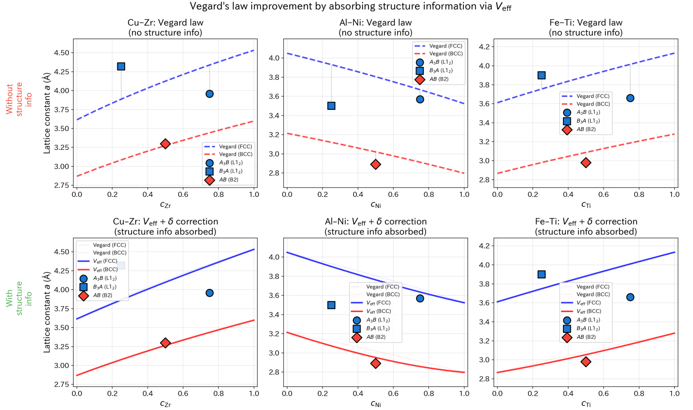
Figure 14: 構造情報吸収による Vegard 則の改善（代表 3 ペア：Cu-Zr, Al-Ni, Fe-Ti）。上段：Vegard 則（純元素体積の線形補間）。赤破線：BCC 予測、青破線：FCC 予測。DFT 計算値（丸： A_3B (L1 2 )、四角： B_3A (L1 2 )、菱形： AB (B2)）は Vegard 直線から系統的に偏差する。下段： V_{\text{eff}} ( \delta^{(s)} 補正後)。赤実線：BCC ( \delta^{B2} 使用)、青実線：FCC ( \delta^{L1_2} 使用)。構造特異的な \delta 補正により Vegard 直線が曲線に変換され、DFT 点に接近する。薄い点線は補正前の Vegard 則。
