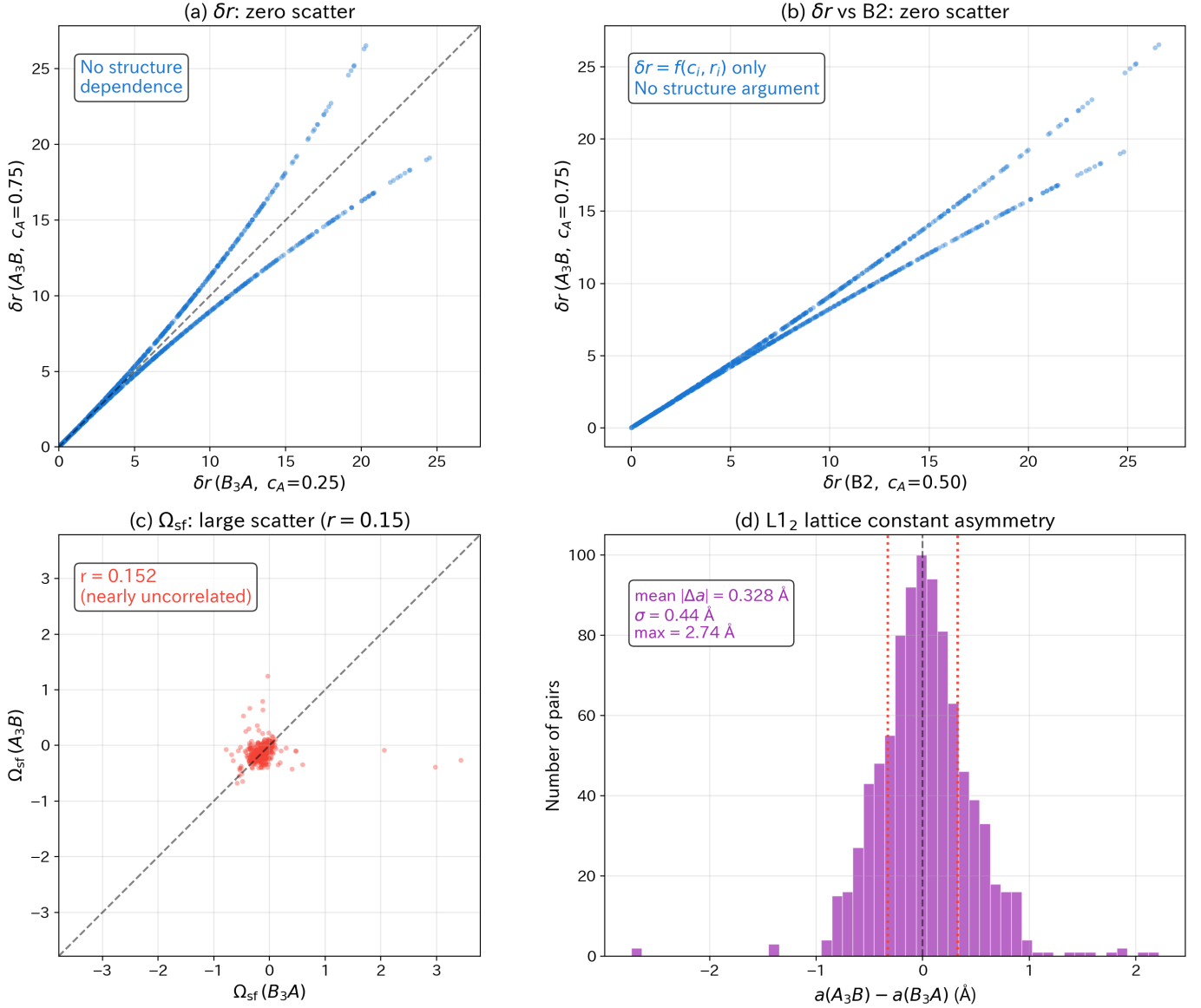
Figure 8: \delta r の構造不変性の証明 (905 二元系ペア)。 (a) \delta r(A_3B) vs \delta r(B_3A) : 散布ゼロ ( \delta r は組成 c と純元素半径 r_i のみの関数であり、構造情報を含まない)。 (b) \delta r(A_3B) vs \delta r(B_2) : 同じく散布なし。 (c) \Omega_{sf}(A_3B) vs \Omega_{sf}(B_3A) : 大きな散布 (相関 r = 0.15 、ほぼ無相関)。 \Omega_{sf} は構造 (配位環境) の情報を内包する。 (d) L1_2 格子定数差 a(A_3B) - a(B_3A) のヒストグラム。平均差 0.328 Å、最大差 2.74 Å に達し、 \delta r ではこの構造非対称性が不可視。
