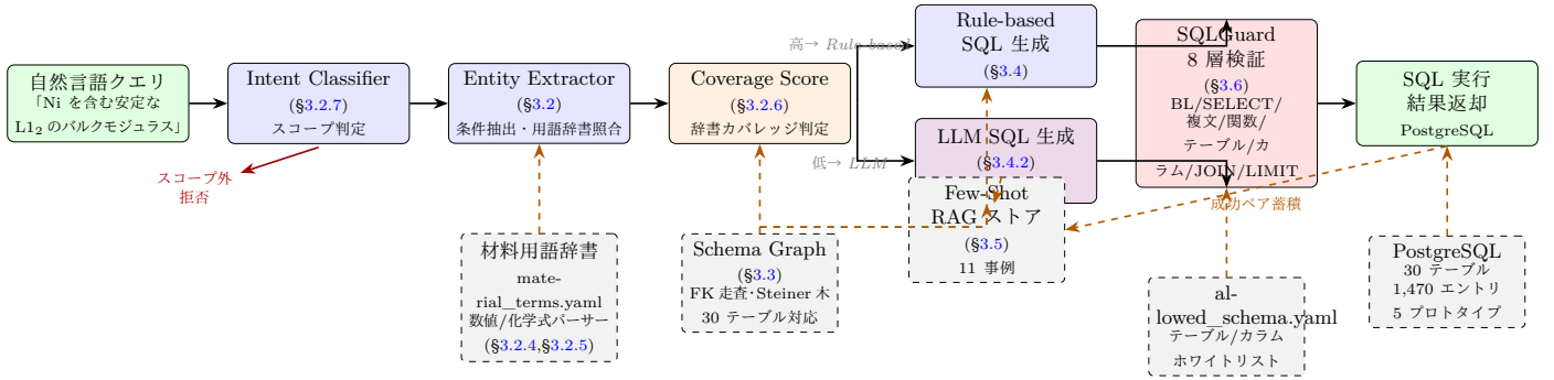
Figure 2: システムアーキテクチャの全体構成。実線矢印は主要データフロー、破線矢印 (橙色) はデータ参照・フィードバックループを示す。Coverage Score に基づき Rule-based (高カバレッジ) または LLM (低カバレッジ) 経路に分岐し、いずれも Schema Graph (30 テーブル FK 走査) による JOIN パス制約と SQLGuard 8 層検証を経て安全な SQL が生成・実行される。実行エラーまたは空結果が検出された場合は、エラー診断情報付きで LLM にリペアを依頼するリペアループ (最大 2 回) が作動する。成功したクエリペヤは Few-Shot RAG ストアに蓄積され、以降の LLM 生成に活用される。
