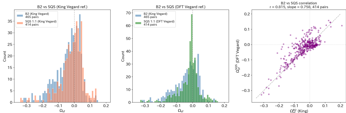
Figure 14: \Omega_{sf} 分布の比較。(左) B2 vs SQS 1:1 (King Vegard 参照)。B2 は負側に偏る。(中) B2 vs SQS 1:1 (DFT Vegard 参照)。DFT 参照でゼロ近傍に集中。(右) B2-SQS 散布図 (DFT Vegard 参照、414 共通ペア)。傾き 0.76。
