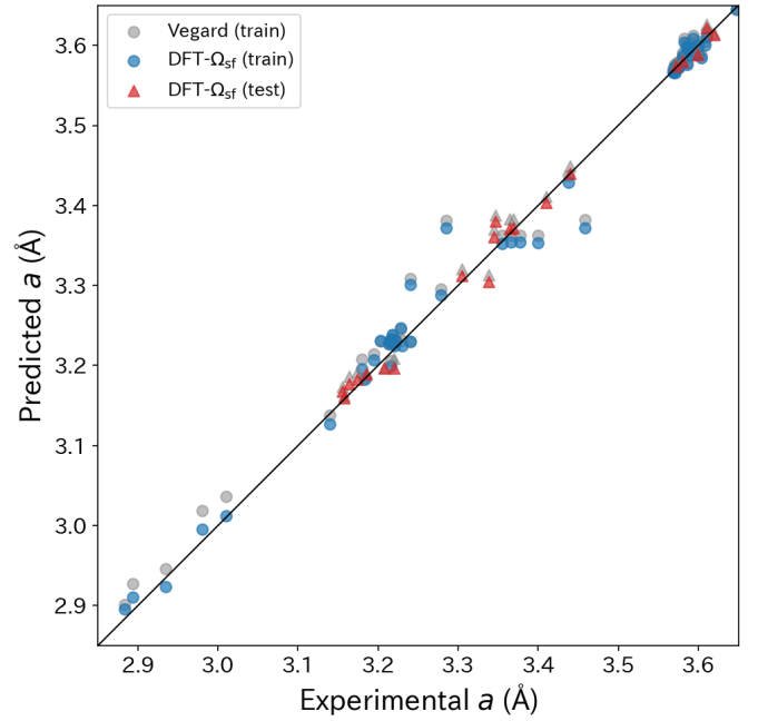
Figure 2: 全 87 HEA のパリティプロット (予測 vs 実験格子定数)。灰色: Vegard 則による予測 (64 HEA 訓練セット)、青色: DFT- \Omega_{\text{sf}} モデルによる予測 (同 64 HEA、RMSE = 0.0214 \text{\AA} )、赤色三角: 独立テストセット (28 HEA、RMSE = 0.0154 \text{\AA} )。対角線は a_{\text{pred}} = a_{\text{exp}} を表す。
