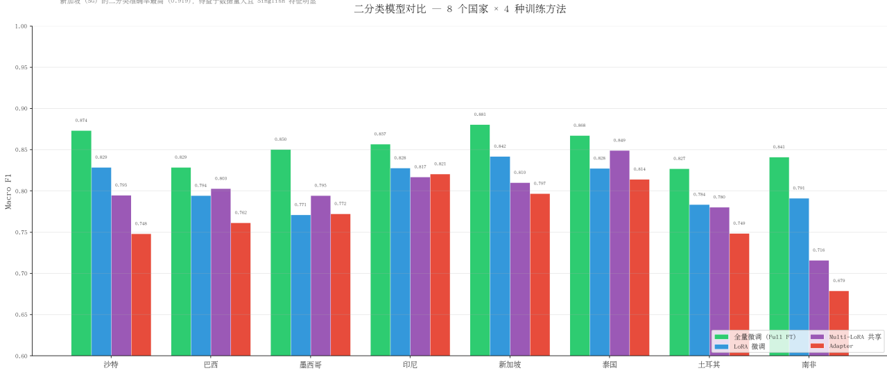
图 1: 8 国 × 4 种方法二分类 Macro F1 对比。全量微调 (绿) 在所有国家都表现最优，平均领先 LoRA +0.044
