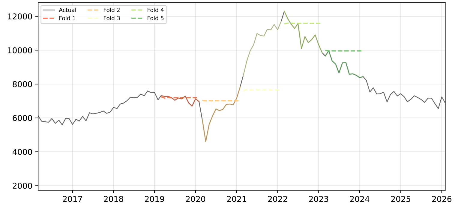
INDPRO | NRMSE h=1: 0.040 h=12: 0.075
