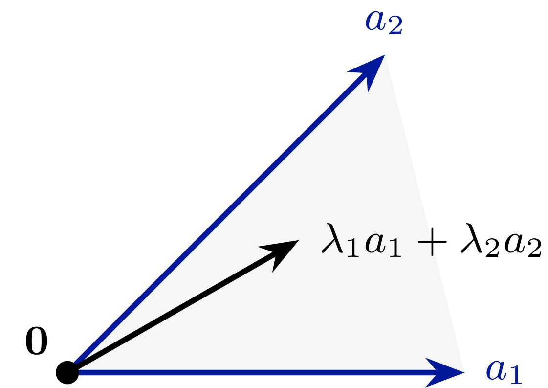
2方向 a_1, a_2 で生成される凸錐
