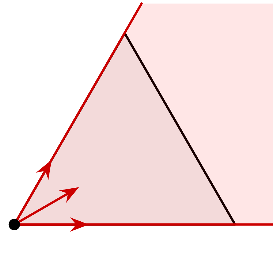
頂点 e_1 h_2, h_3 \geq 0 \ (h \in L)
