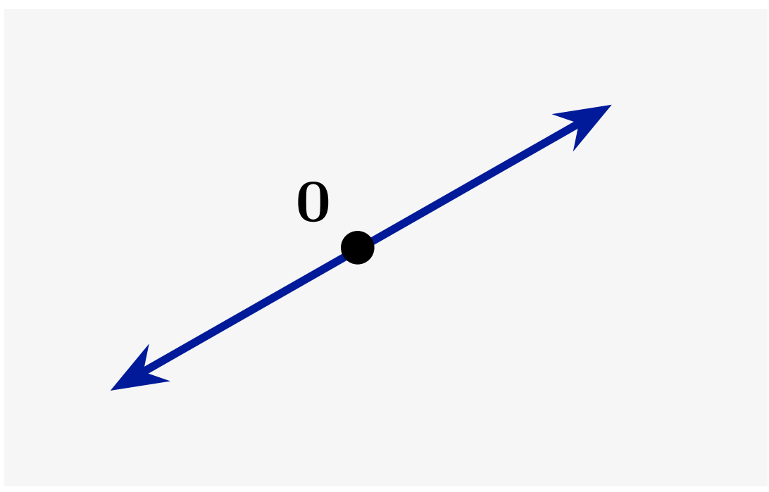
線形空間も錐
