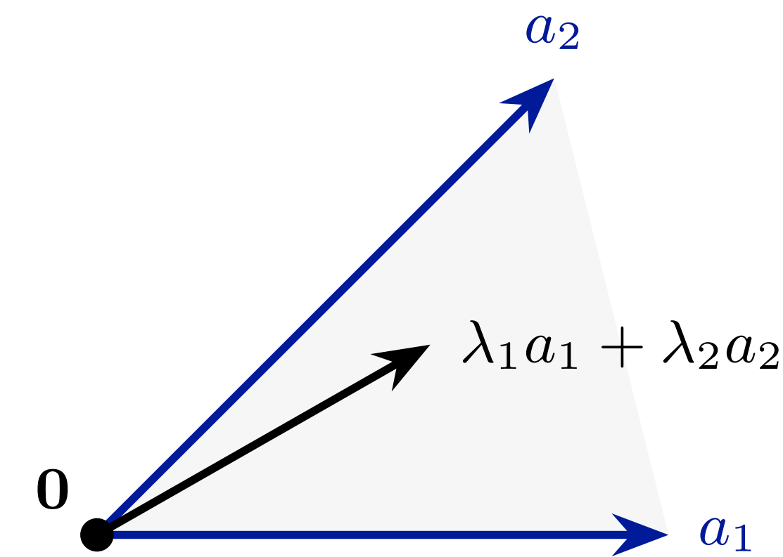
2方向 a_1, a_2 で生成される凸錐
