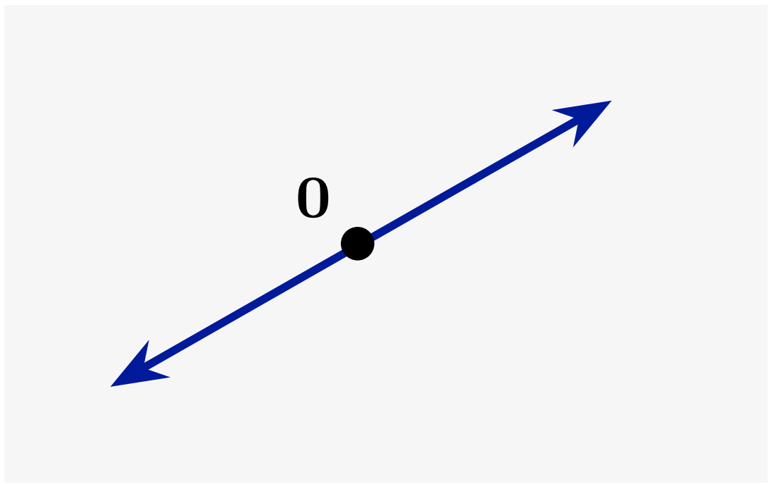
線形空間も錐
