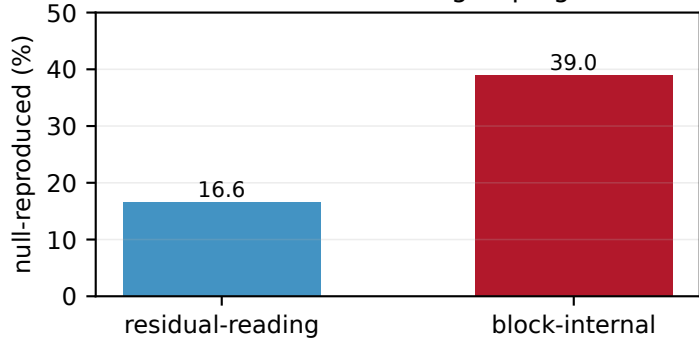
ViT-B/16 module grouping
