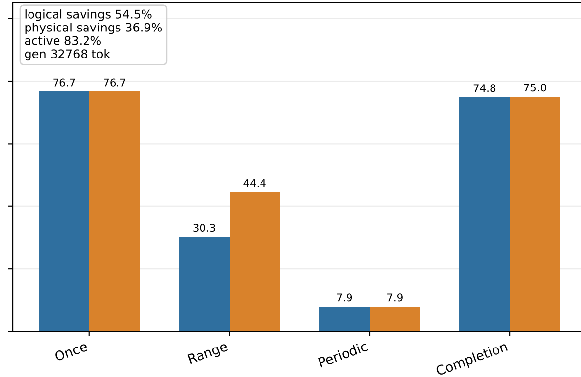
SGT long
