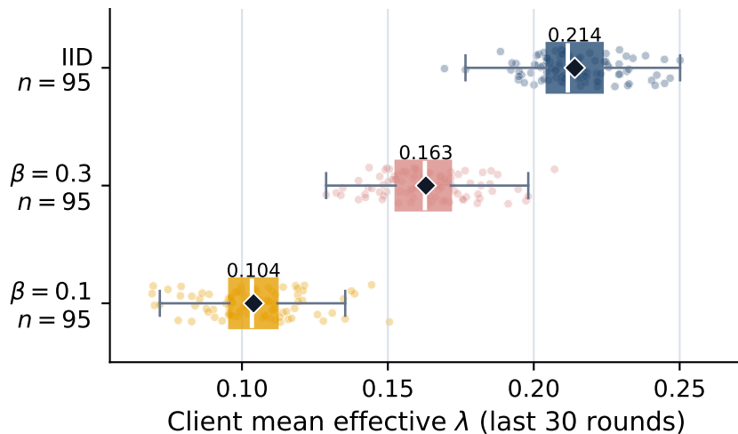
TinyImageNet
