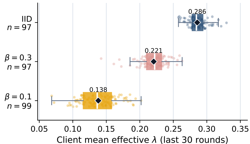
ImageNet100-64
