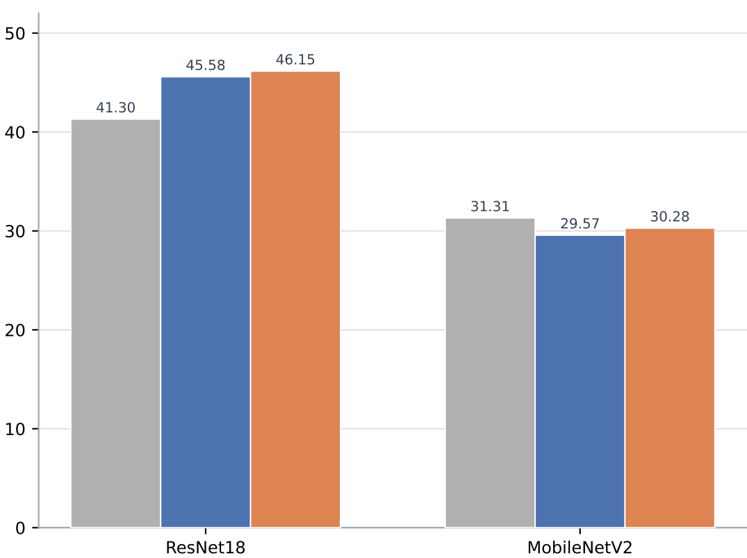
TinyImageNet
