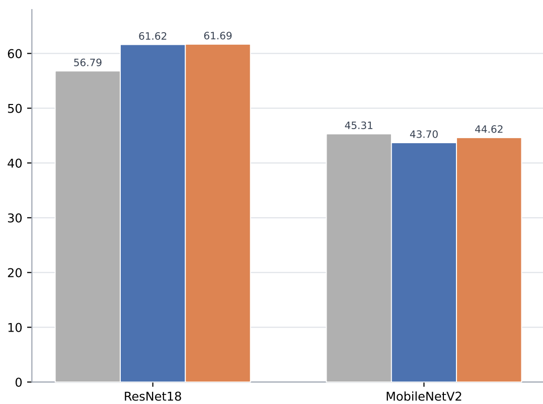
ImageNet100-64
