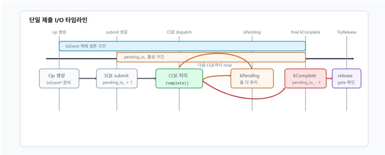
그림 2.2: ioevent lifetime
