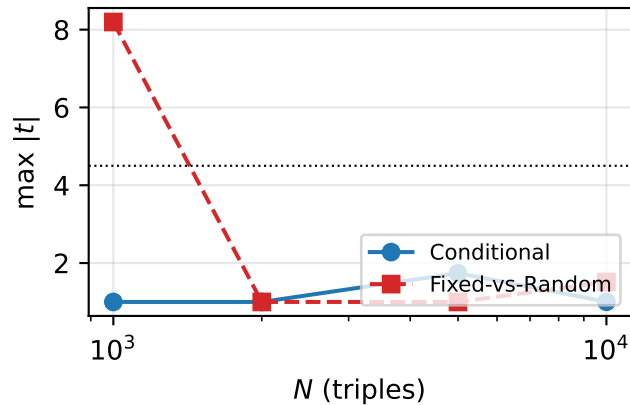
TVLA max |t| (order 1)
