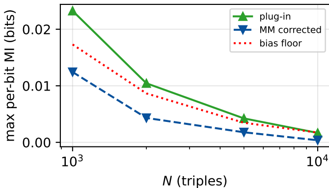
(d) per-bit MI on power trace ( d = 2 )
