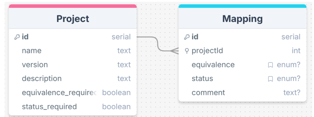
Ausschnitt aus Datenbankschema
