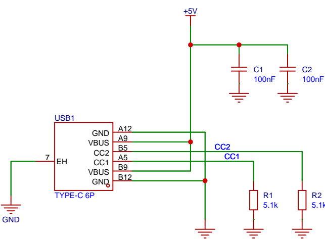
USB-C(INPUT)
