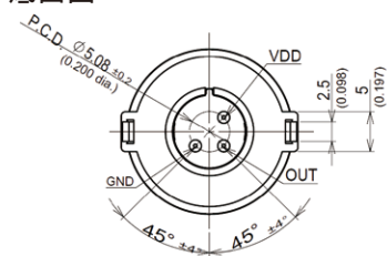
底面図
