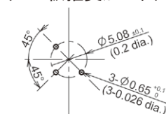
プリント板推奨加工図
