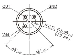
外形寸法図
